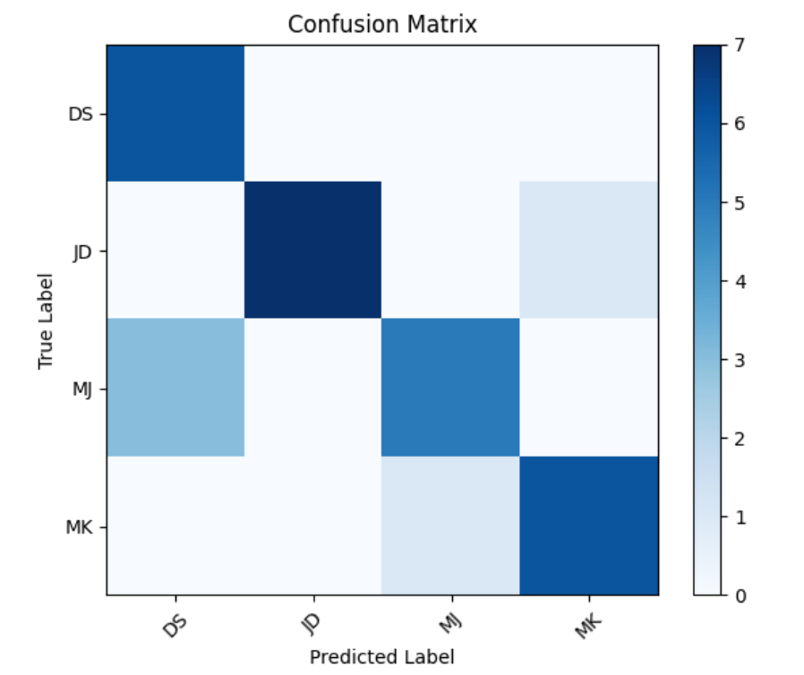
Rysunek 6.2: Wykres przedstawiający macierz konfuzji klasyfikatora danych oczyszczonych dla 4 klas
