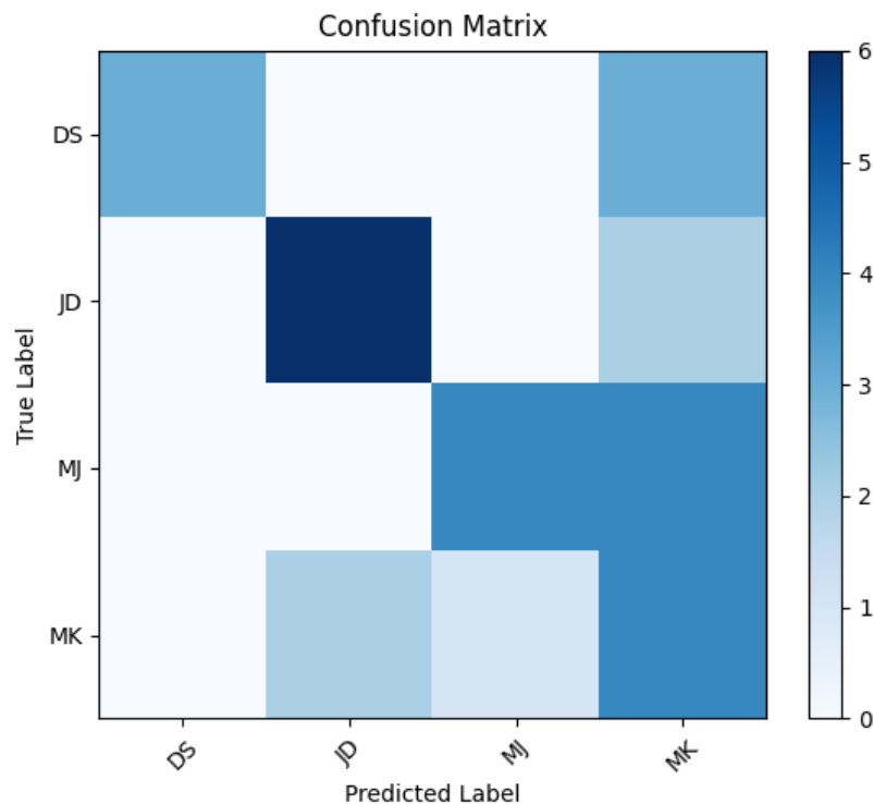
Rysunek 6.3: Wykres przedstawiający macierz konfuzji klasyfikatora danych surowych dla 4 klas
