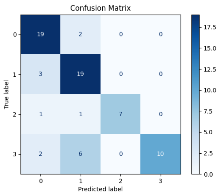
Rysunek 6.5: Wykres przedstawiający macierz konfuzji klasyfikatora NN dla 4 klas
