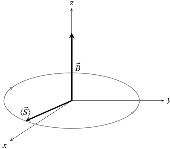
Gambar 1: Evolusi waktu dari \langle \vec{S} \rangle untuk partikel spin-1/2 (contohnya sebuah proton) di dalam medan magnet statis.
