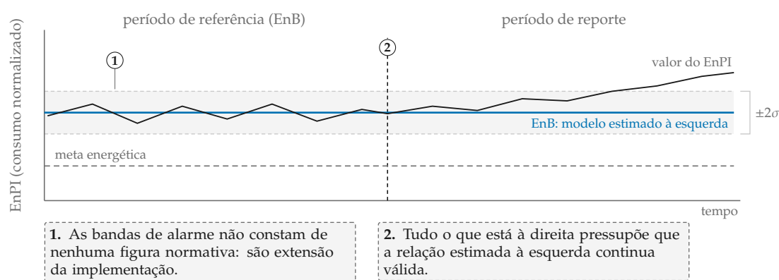
Figura 2.2: O conceito EnPI/EnB/meta e a fronteira entre o que a norma desenha e o que a implementação acrescenta. A comparação entre o valor do indicador e a referência é o mecanismo que a ISO 50001 exige (§9.1.1); a banda de alarme em torno da referência não aparece em nenhuma figura normativa e é escolha da organização. O Anexo D da ISO 50006 usa o modelo estimado no período de referência para prever o período de reporte e lê a diferença como melhoria de desempenho, sem enunciar a transportabilidade da relação como pressuposto. Esquema próprio, sem dados, a partir de [83, 58].
