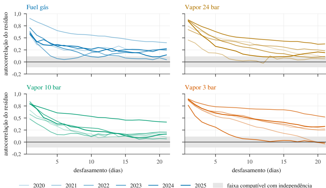
Figura 6.3: Autocorrelação dos resíduos das regressões oficiais, por vetor e por ano completo, até 21 dias de defasamento. A cor identifica o vetor e o tom identifica o ano, do mais claro (2020) ao mais escuro (2025). A faixa cinzenta é o intervalo em que a autocorrelação seria compatível com independência ao nível de 5 %, dado o número de pares disponíveis em cada defasamento. Nenhum vetor, em nenhum ano, tem resíduos compatíveis com independência à escala do dia, e nos vapores a dependência estende-se a duas e três semanas. É esta a razão pela qual os erros-padrão e os p -values clássicos não são usados neste capítulo e toda a incerteza é estimada por reamostragem em blocos.
