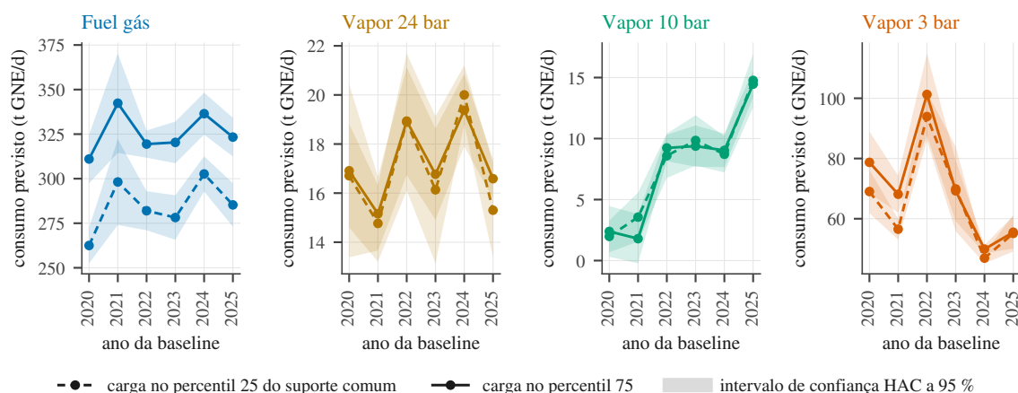
Figura 6.5: Consumo previsto por cada baseline anual, avaliado em duas cargas fixas dentro do suporte comum a todos os anos — os percentis 25 e 75 da carga observada — com o intervalo de confiança a 95 % construído com erros-padrão robustos a heterocedasticidade e autocorrelação. A comparação faz-se aqui, e não no intercepto: o valor da reta em Q = 0 está fora do domínio observado e não é um consumo base físico. A rejeição estatística da hipótese de coeficientes constantes ao longo dos anos é sensível ao tratamento da dependência temporal, como o Apêndice C documenta.
