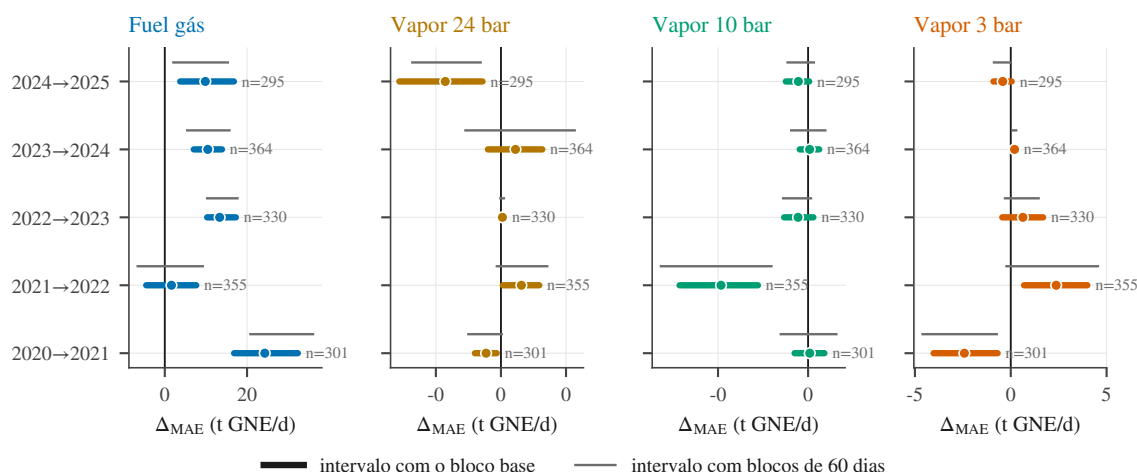
Figura 6.4: Diferença de erro absoluto médio entre a baseline e o nulo trivial — a média do ano de treino — em cada transição treino → teste. Valores à direita da linha zero significam que o modelo erra menos do que o nulo. O traço grosso é o intervalo de confiança a 95 % com o comprimento de bloco base; o traço fino, deslocado, é o mesmo intervalo com blocos de 60 dias, e a distância entre os dois é a medida honesta da sensibilidade a essa escolha. O n anotado é o número de dias avaliados, comum ao modelo e ao nulo. Só o fuel gás tem ganho que exclui o zero na maioria das transições; nos três vapores há transições em que o nulo é melhor.
