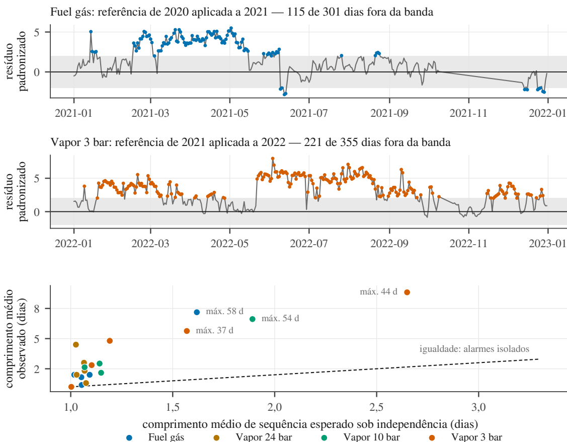
Figura 6.7: Os alarmes não chegam isolados. Em cima, os resíduos padronizados dos dois casos mais extremos, dia a dia, com a banda de produção — dois desvios-padrão do ano de treino — a cinzento e os dias em alarme assinalados; a reconstrução a partir dos parâmetros oficiais reproduz exatamente as contagens da corrida canônica, 115 em 301 e 221 em 355. Em baixo, o comprimento médio das sequências de dias consecutivos em alarme, observado contra o que se esperaria se cada dia em alarme fosse independente do anterior, para todos os vetores e transições. Todos os pontos estão acima da diagonal e os casos com mais alarmes estão muito acima dela: uma sequência de 44 ou de 58 dias consecutivos não é um dia anômalo, é um período inteiro em que a referência deixou de descrever a unidade. Os comprimentos de sequência são descritivos e não sustentam, por si, um teste de independência.
