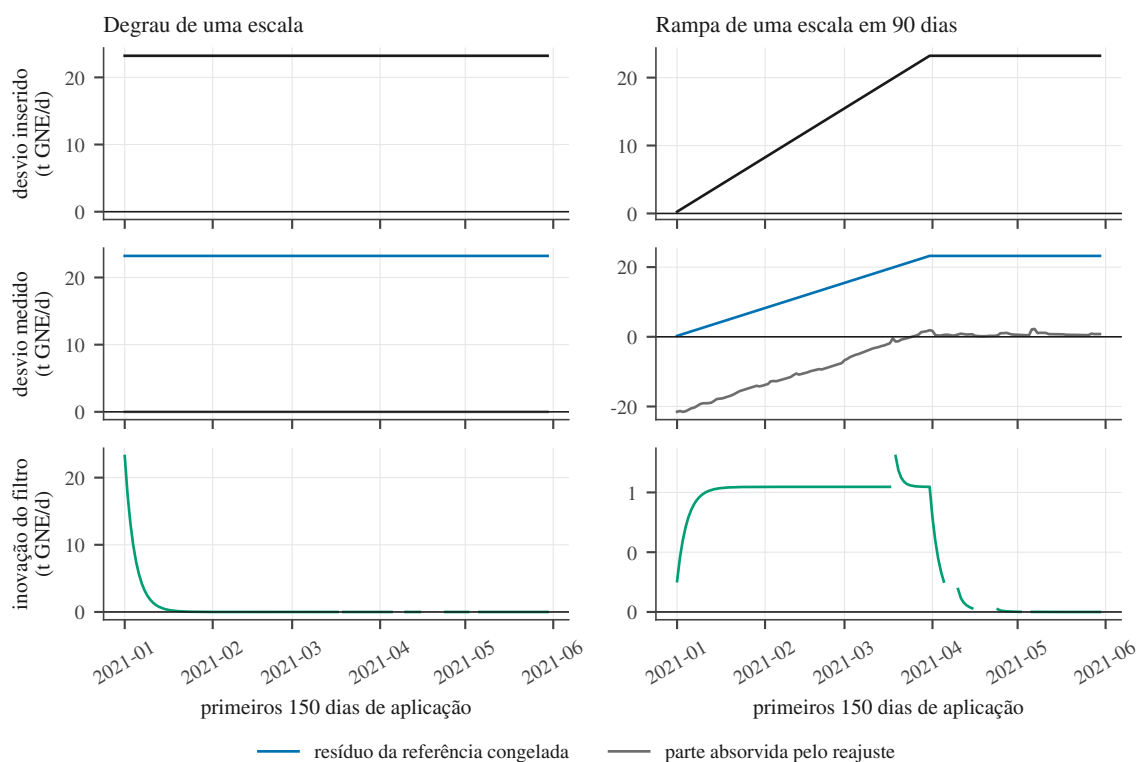
Figura 7.3: Experiência de injeção no fuel gás: um desvio conhecido é somado à série e segue-se o que resta dele em cada componente, nos primeiros 150 dias de aplicação, para um degrau e para uma rampa da mesma amplitude. Em cima, o desvio inserido. Ao meio, o desvio medido contra a referência congelada e a parte que o reajuste anual absorve. Em baixo, a inovação do filtro. A diferença entre os dois primeiros painéis é uma identidade algébrica, não uma medição; o terceiro painel é que mostra a atenuação efetiva. Os valores numéricos citados no texto vêm do lote validado, não desta ilustração.
