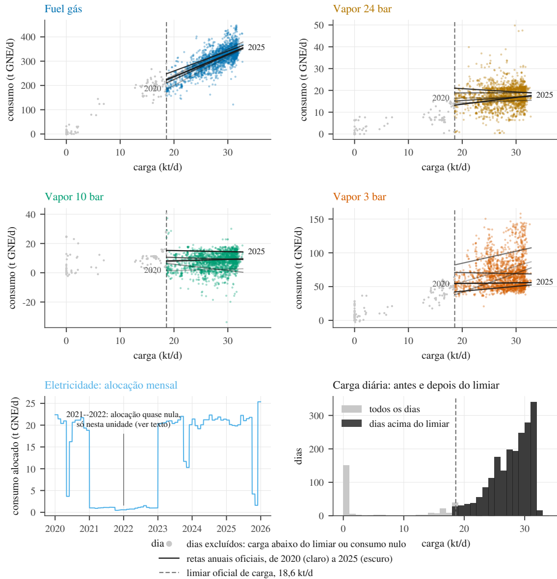
Figura 6.2: Consumo diário contra carga diária, por vetor, na unidade de destilação atmosférica, de 2020 a 2025. Os pontos a cinzento são os dias excluídos — carga abaixo do limiar oficial de 18,6 kt/d ou consumo nulo — e estão desenhados para que a população não coberta pela baseline fique visível. As retas são as regressões anuais oficiais, da mais clara (2020) à mais escura (2025). O painel da eletricidade não é uma dispersão: mostra a série no tempo, e os patamares mensais são o efeito da alocação, não variação de consumo; a quase anulação da alocação em 2021 e 2022, que não se observa em nenhuma outra unidade, está assinalada e discutida no texto. O último painel compara a distribuição da carga diária antes e depois do limiar.
