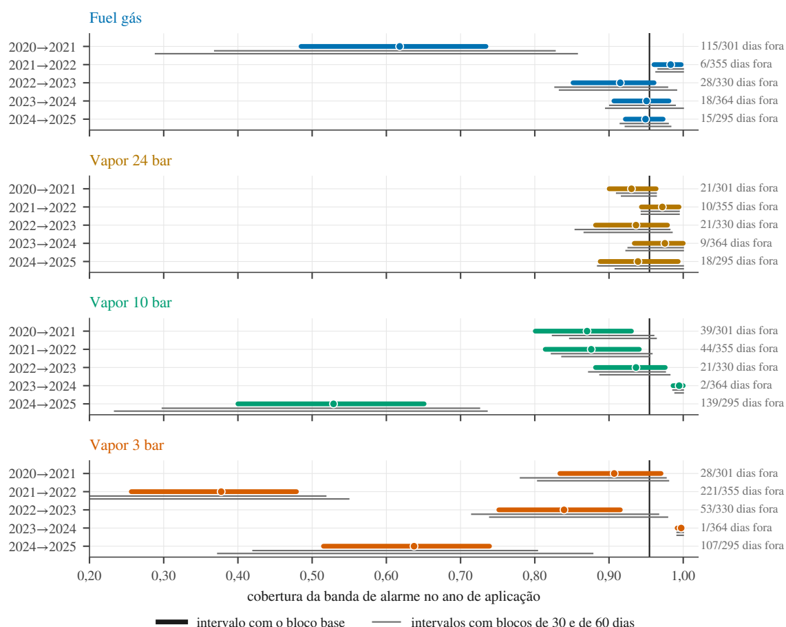
Figura 6.6: Fração de dias do ano de aplicação que caem dentro da banda de alarme construída no ano de treino, por vetor e por transição. A linha vertical é o nível nominal de 0,9545, o que a banda promete. O traço grosso é o intervalo obtido por reamostragem em blocos com o comprimento base; os traços finos, deslocados, repetem o exercício com blocos de 30 e de 60 dias. Um intervalo que inclui o valor nominal não certifica a banda: apenas diz que os dados disponíveis não a excluem. A contagem à direita dá os dias fora da banda sobre os dias avaliados.
