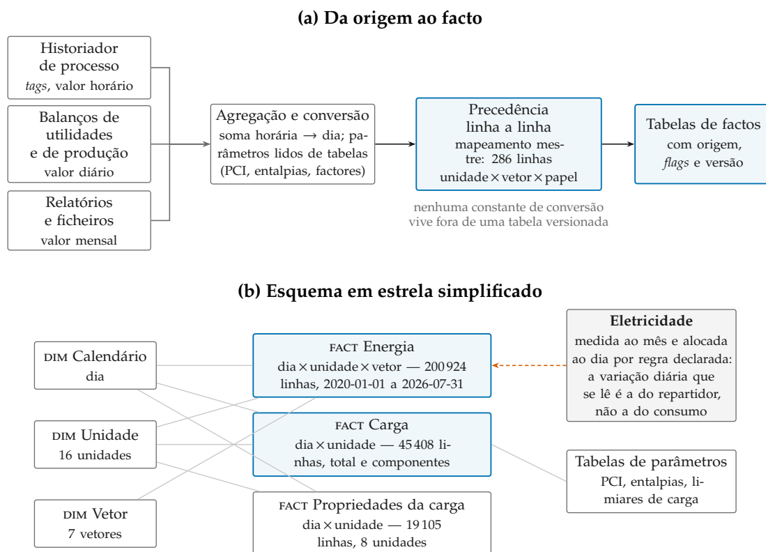
Figura 4.1: Arquitetura de dados da plataforma. No painel (a), o percurso de cada valor desde a origem até ao facto: a agregação e a conversão usam parâmetros lidos de tabelas, e a escolha entre canais é resolvida linha a linha pelo mapeamento mestre, não por código. No painel (b), o esquema em estrela reduzido às três tabelas de factos e às três dimensões que este trabalho usa, com a granularidade de cada facto escrita por extenso. A eletricidade é a única exceção à granularidade diária: é medida ao mês e alocada ao dia por uma regra declarada, pelo que a variação diária que dela se lê não é variação de consumo. O modelo completo tem 32 tabelas e está descrito no dicionário de dados (Apêndice D).
