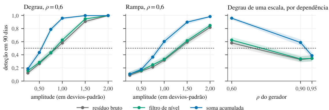
Figura 7.4: Probabilidade de detetar um desvio nos primeiros 90 dias, por amplitude, para três monitores calibrados ao mesmo orçamento de falsos sinais. Os dois primeiros painéis separam degrau de rampa com dependência moderada ( \rho = 0,6 ); o terceiro fixa a amplitude num desvio-padrão e varia a dependência do gerador. A banda é o intervalo de Wilson sobre as réplicas. A linha a tracejado marca metade das deteções. Os valores descrevem o gerador simulado e as suas hipóteses, e não são uma previsão do que aconteceria na refinaria.
