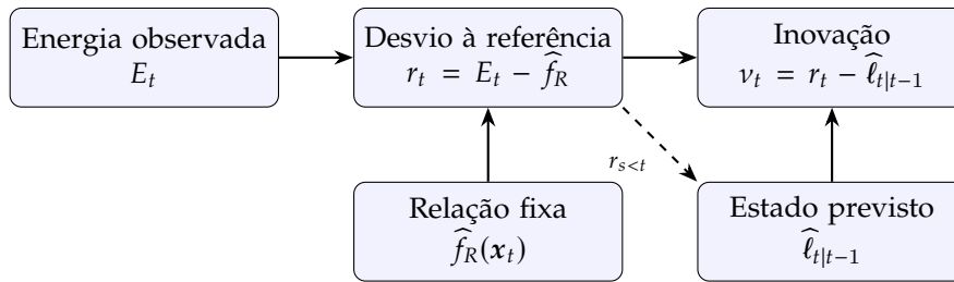
Figura E.2: Decomposição conceitual dos canais. O estado previsto é calculado a partir dos desvios anteriores; a atualização com r_t só afeta previsões posteriores.
