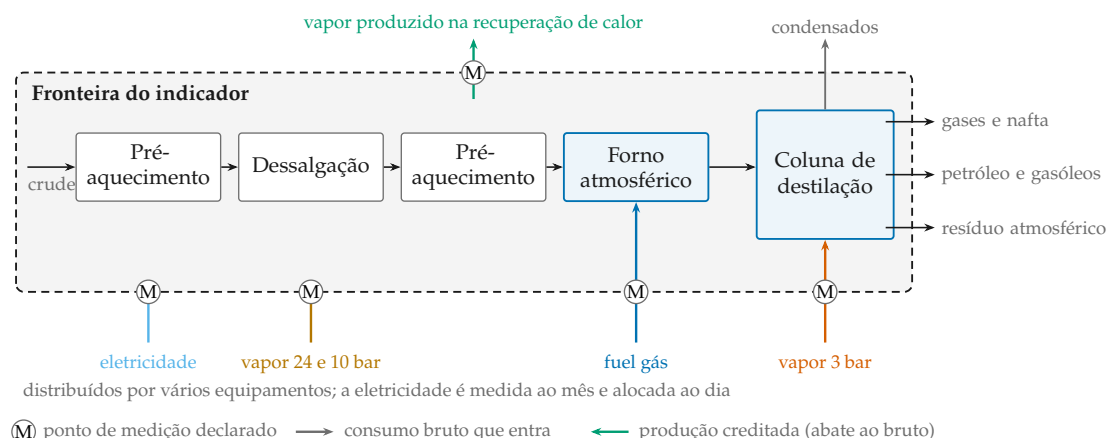
Figura 2.3: Esquema funcional da unidade de destilação atmosférica e da fronteira que o indicador de desempenho usa. O desenho não tem escala nem caudais: representa a sequência de operações e os pontos onde entra e sai energia. Três noções de consumo convivem e não devem ser confundidas: o consumo bruto é tudo o que atravessa a fronteira para dentro; o consumo líquido desconta a produção creditada, como o vapor gerado na recuperação de calor; o consumo alocado reparte por unidade aquilo que é medido num ponto comum, segundo uma regra declarada — é o caso da eletricidade, medida ao mês para um conjunto de equipamentos e repartida por dia. Por isso, um desvio medido nesta fronteira pode ter origem no processo ou na regra de repartição.
