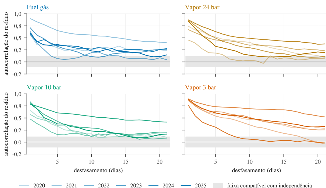
Figura 6.3: Autocorrelação dos resíduos das regressões oficiais, por vetor e por ano completo, até 21 dias de desfasamento. A cor identifica o vetor e o tom identifica o ano, do mais claro (2020) ao mais escuro (2025). A faixa cinzenta é o intervalo em que a autocorrelação seria compatível com independência ao nível de 5 %, dado o número de pares disponíveis em cada desfasamento. Nenhum vetor, em nenhum ano, tem resíduos compatíveis com independência à escala do dia, e nos vapores a dependência estende-se a duas e três semanas. É esta a razão pela qual os erros-padrão e os p -values clássicos não são usados neste capítulo e toda a incerteza é estimada por reamostragem em blocos.
