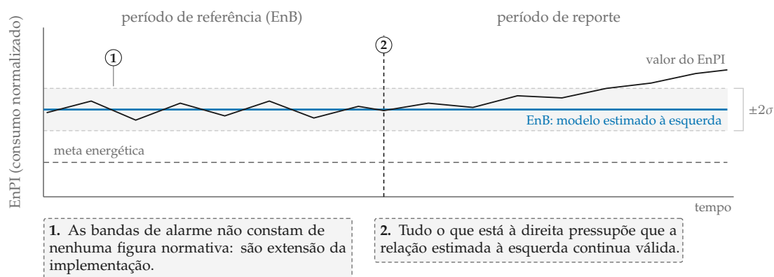
Figura 2.2: O conceito EnPI/EnB/meta e a fronteira entre o que a norma desenha e o que a implementação acrescenta. A comparação entre o valor do indicador e a referência é o mecanismo que a ISO 50001 exige (§9.1.1); a banda de alarme em torno da referência não aparece em nenhuma figura normativa e é escolha da organização. O Anexo D da ISO 50006 usa o modelo estimado no período de referência para prever o período de reporte e lê a diferença como melhoria de desempenho, sem enunciar a transportabilidade da relação como pressuposto. Esquema próprio, sem dados, a partir de [83, 58].
