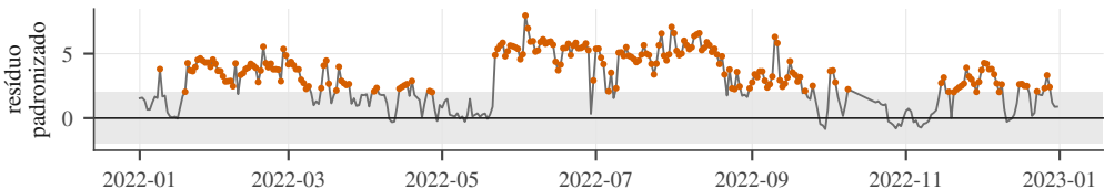
Vapor 3 bar: referência de 2021 aplicada a 2022 — 221 de 355 dias fora da banda
