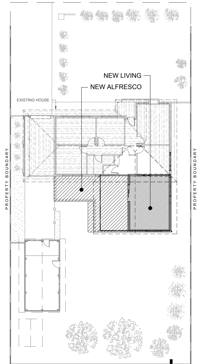
SITE PLAN 1:200
