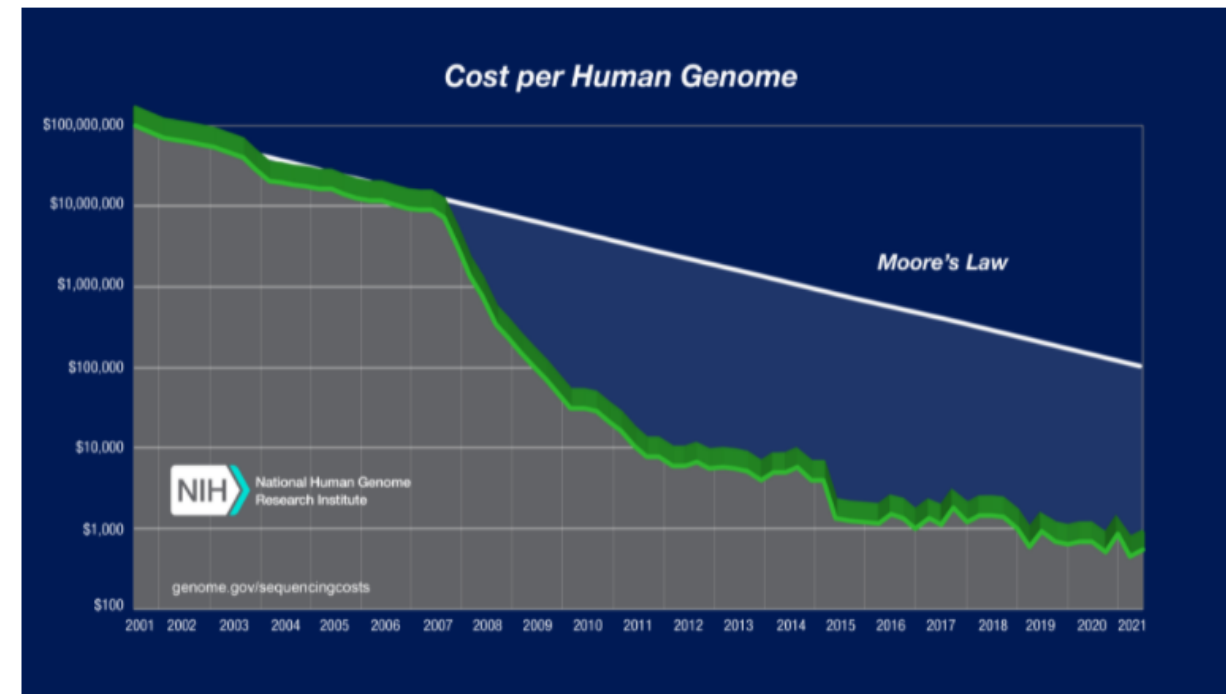
Cost per genome data - 2021
