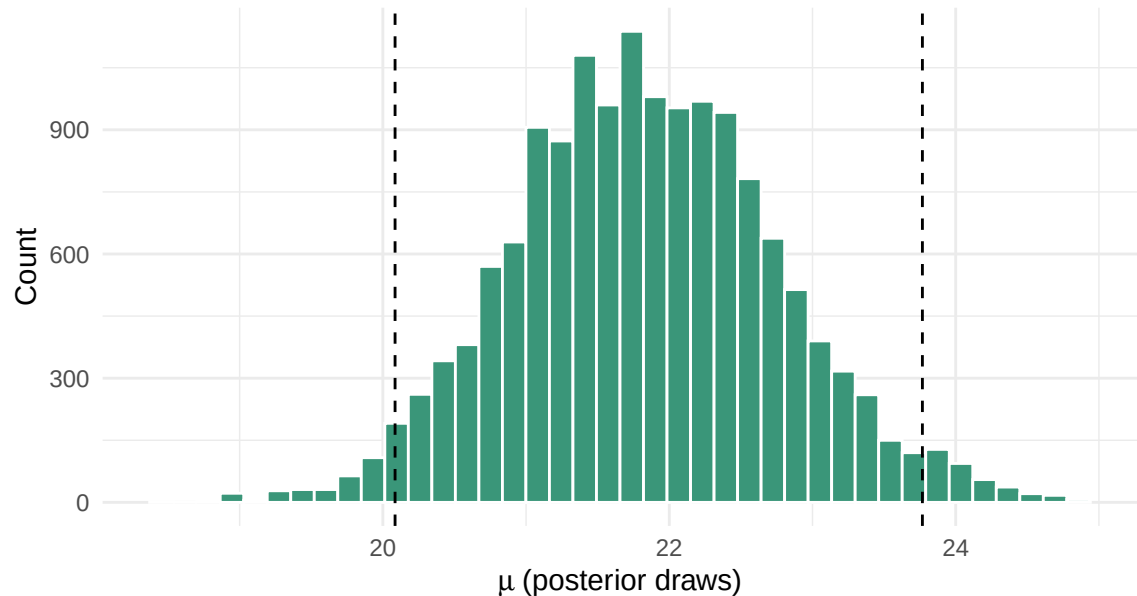
Posterior distribution of \mu
