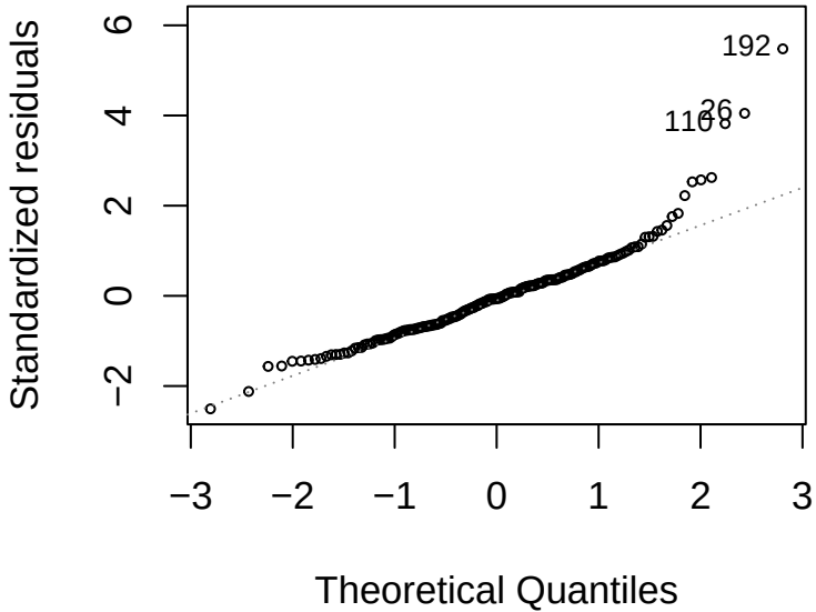
Raw: y \sim x
