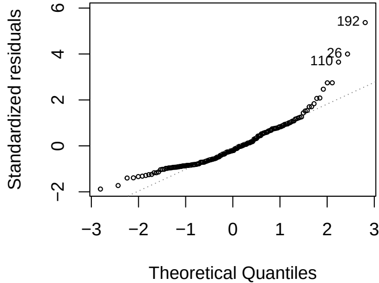
\log(x) : y \sim \log(x)
