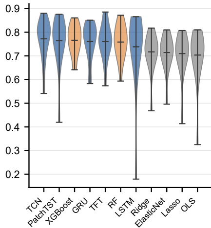
R^2
