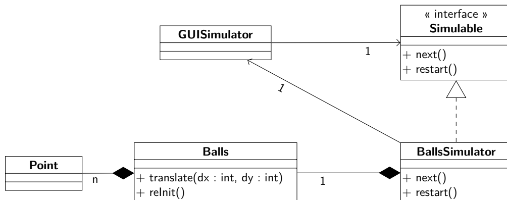
FIGURE 2 – Diagramme des classes permettant de contrôler le simulateur Balls à l'aide de l'interface graphique fournie. La classe BallsSimulator doit réaliser l'interface Simulable , et donc (re)définir les deux méthodes next() et restart() .
