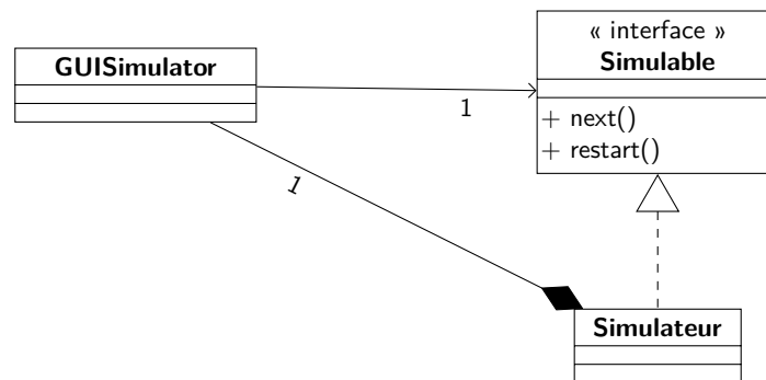
FIGURE 1 – Relation entre l'interface de simulation fournie et le simulateur
