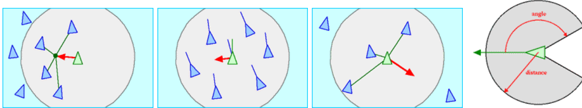
FIGURE 9 – Illustration des principales règles régissant les mouvements de boids . De gauche à droite : cohésion, alignement et séparation. A droite : notion de voisinage, en fonction d'une distance et de l'orientation. Figures issues de la page de Craig Reynolds http://www.red3d.com/cwr/boids/
