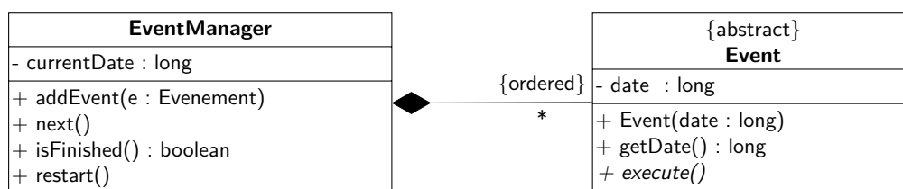
FIGURE 10 – Diagramme de classes d'un gestionnaire à événements discrets
