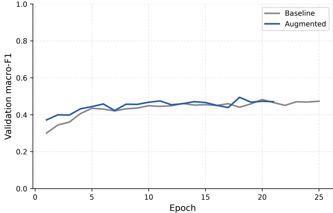
Validation macro-F1
