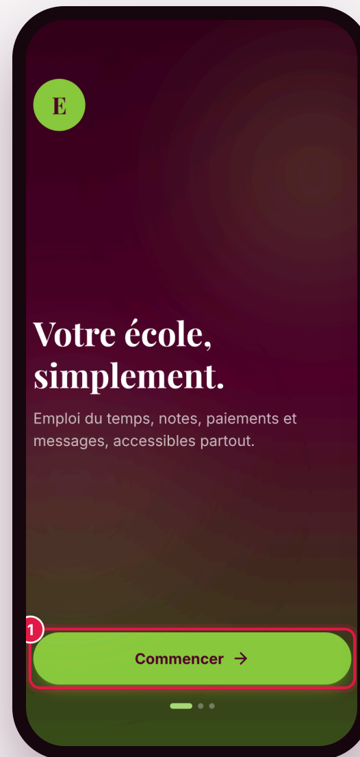
Écran d'accueil
