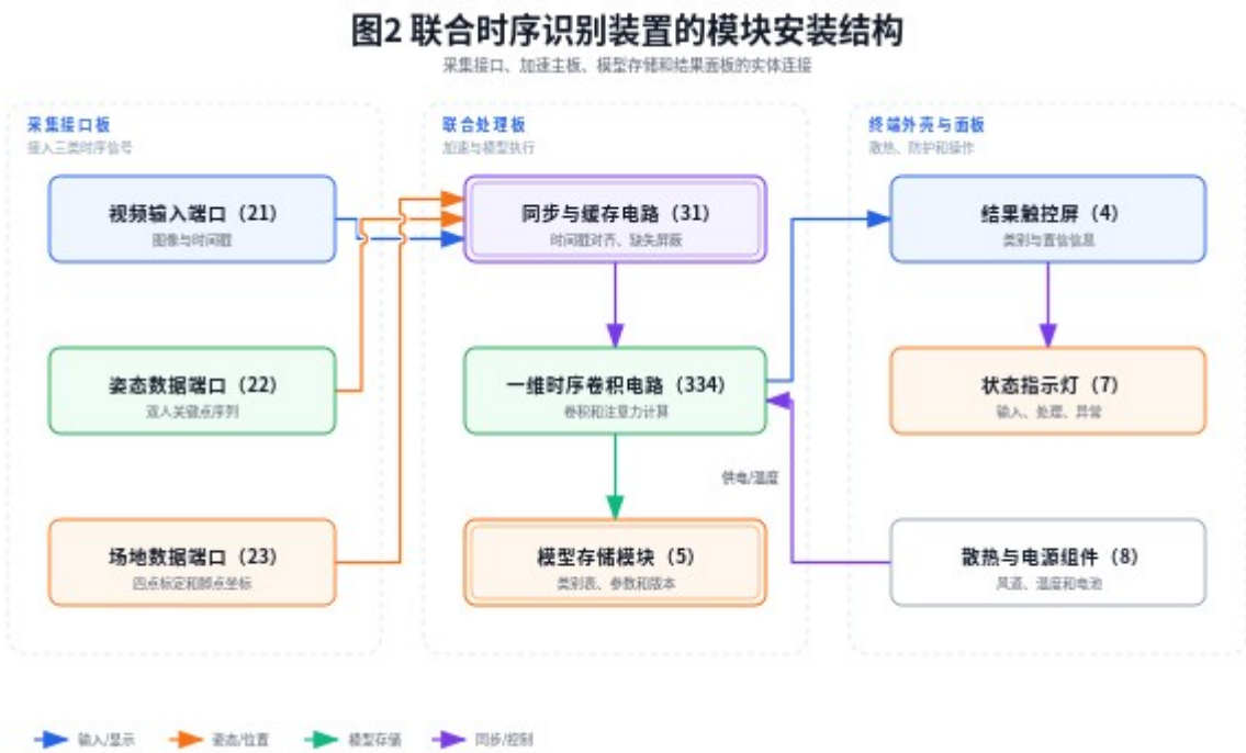
图2 联合时序识别装置的模块安装结构
