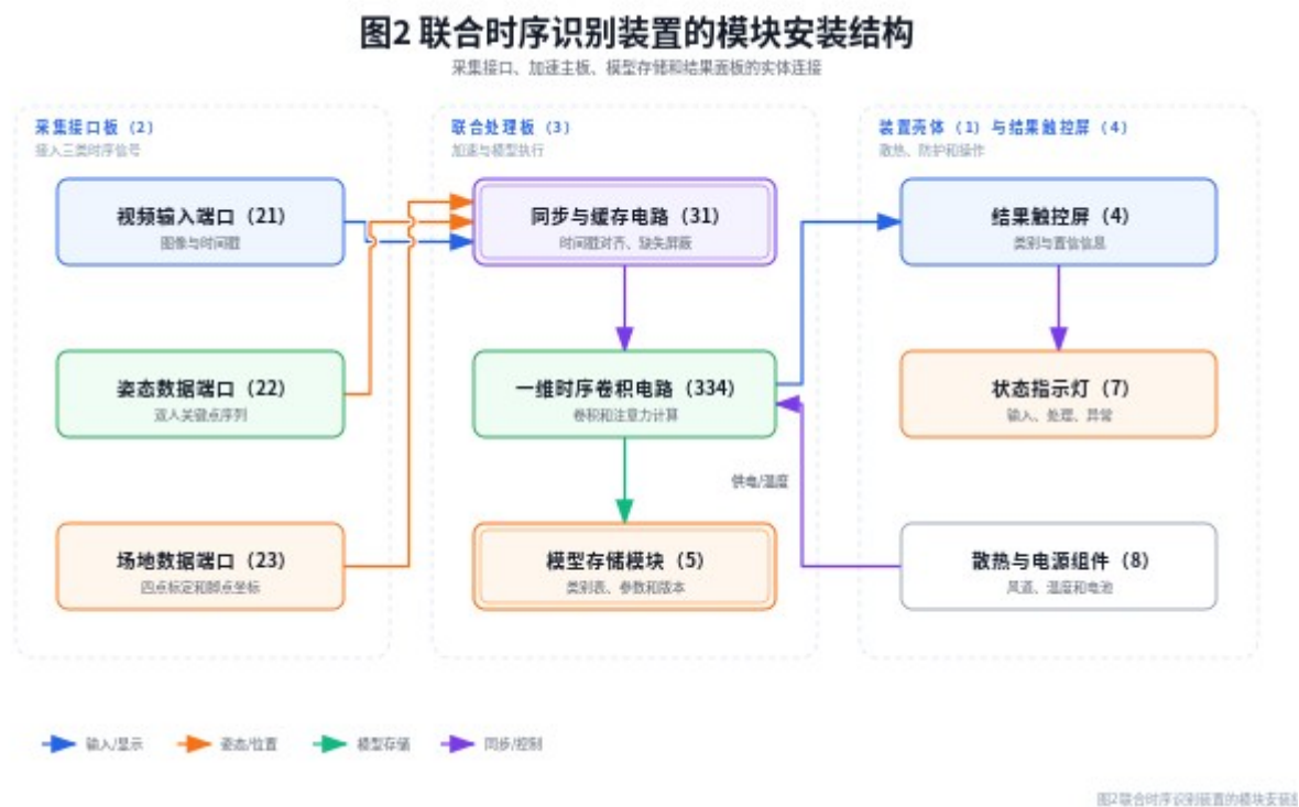
图 2 联合时序识别装置的模块安装结构
