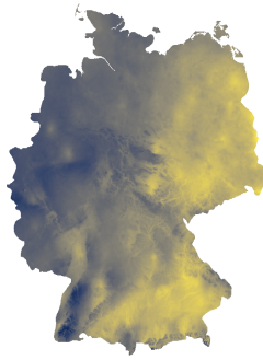
PC2
