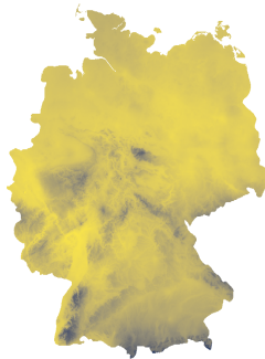
PC2
