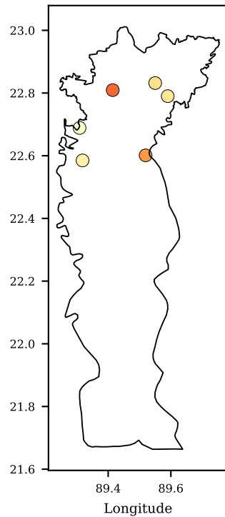
CatBoost
