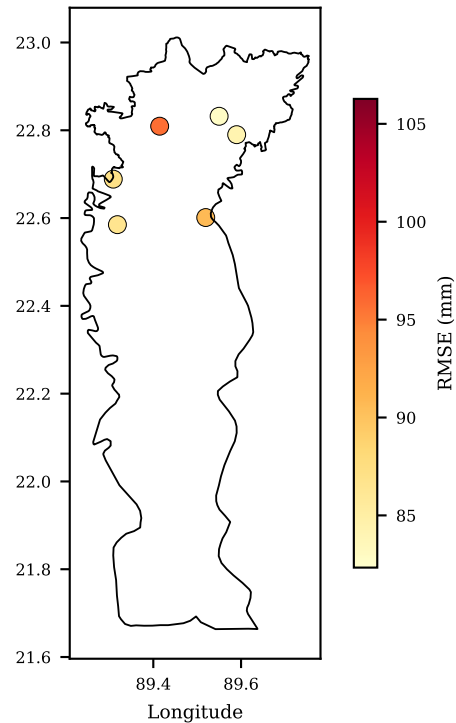
CatBoost
