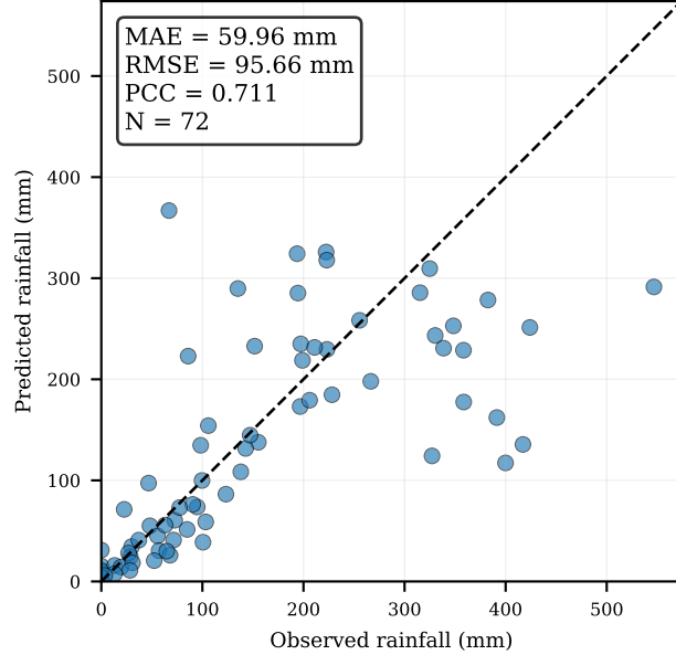
CatBoost
