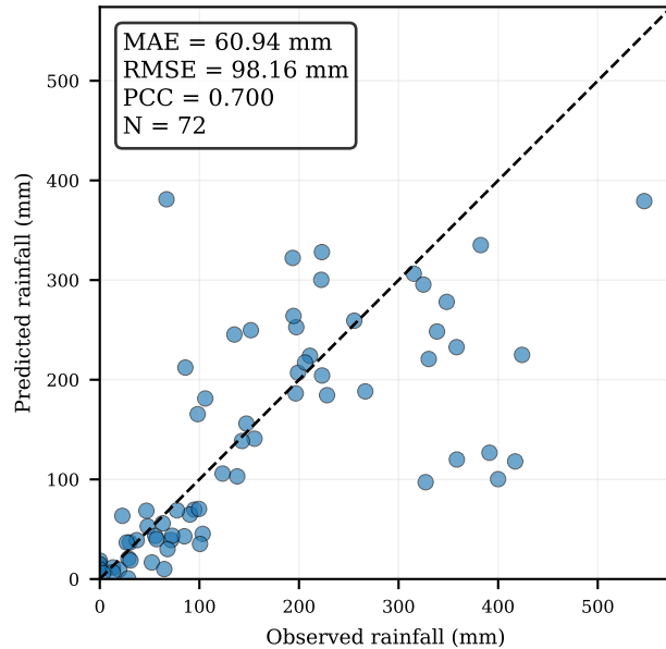
CatBoost
