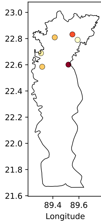
CatBoost
