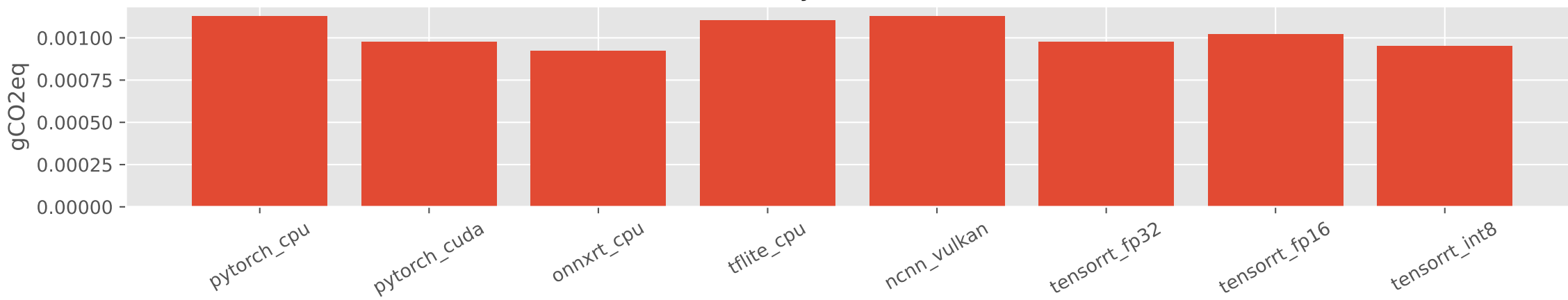
yolov8n
