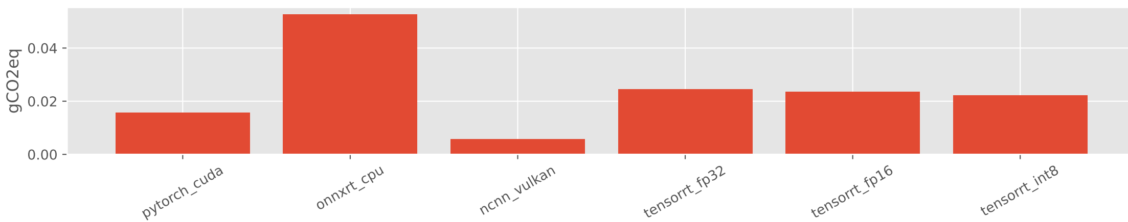
mobilenetv3s
