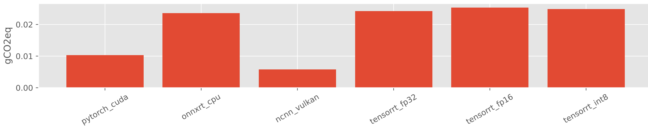
ssd_mv2
