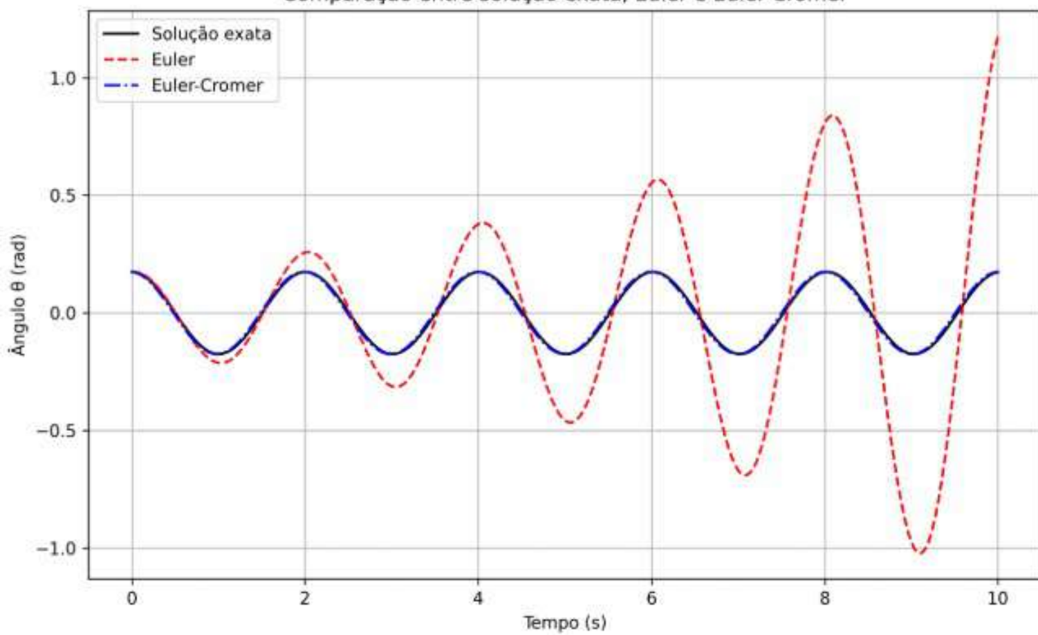
Comparação entre solução exata, Euler e Euler-Cromer
