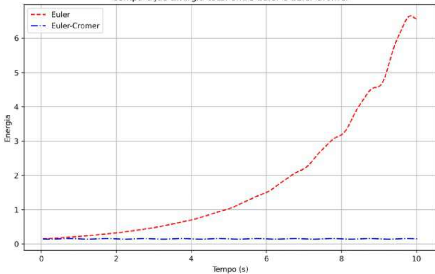
Comparação Energia total entre Euler e Euler-Cromer
