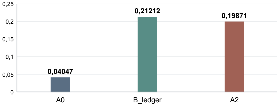
Расходы API, USD
