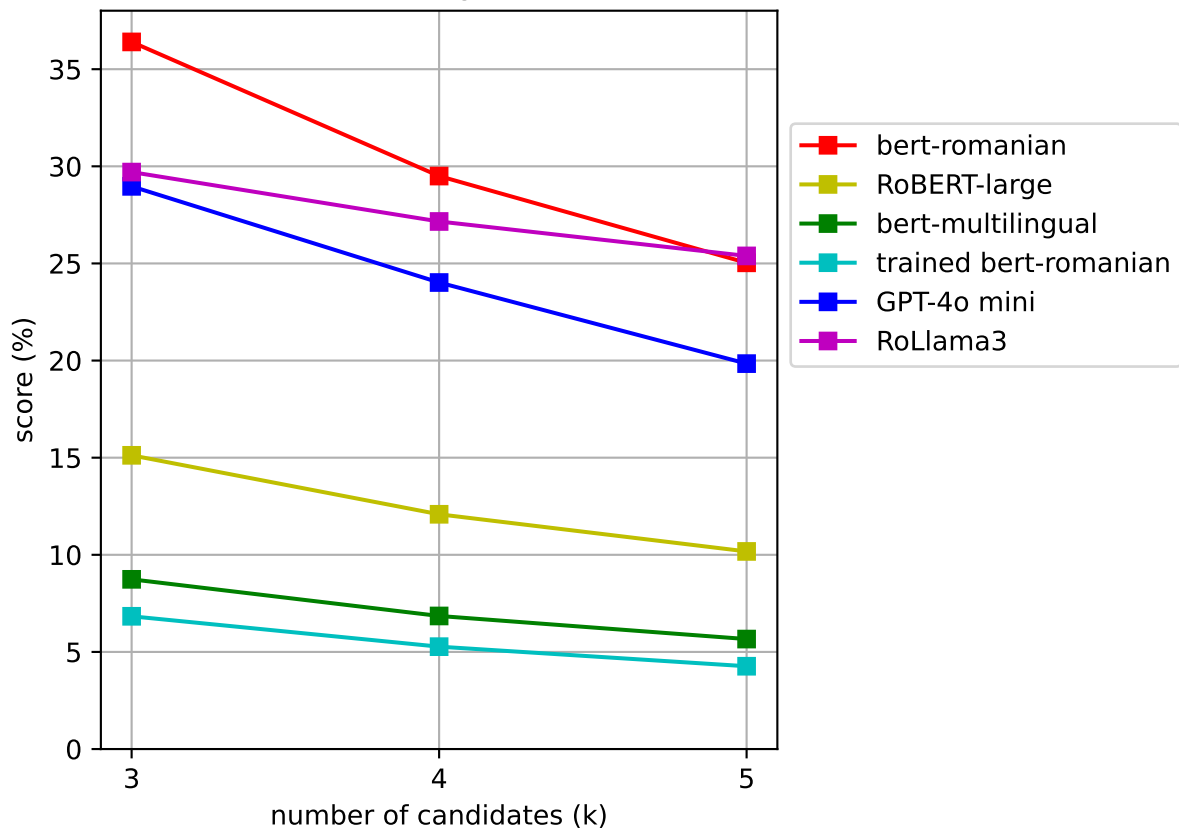
MAP@k
