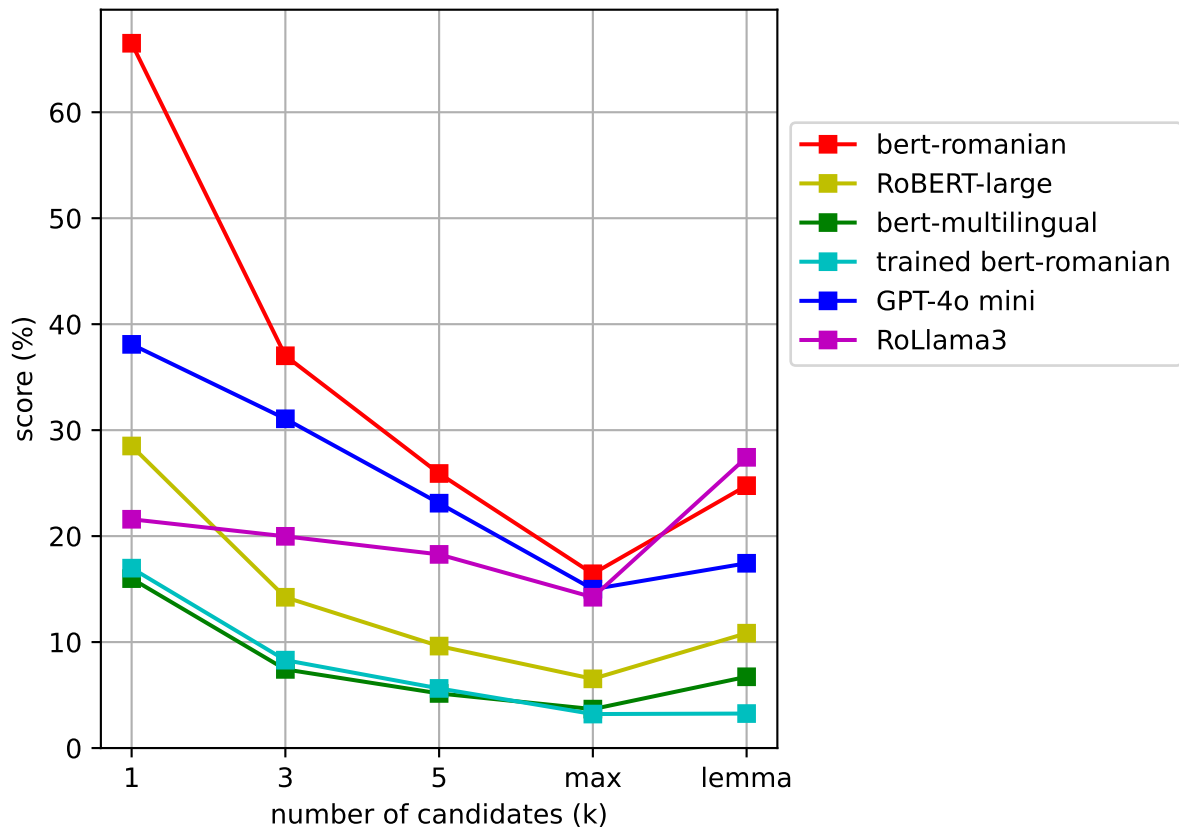
Precision@k
