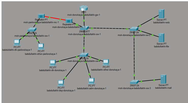
Рис. 8: Схема с повторителями
