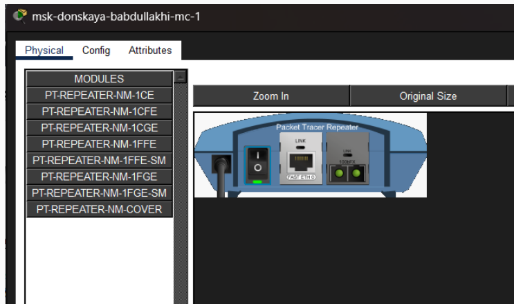
Рис. 7: Настройка повторителей
