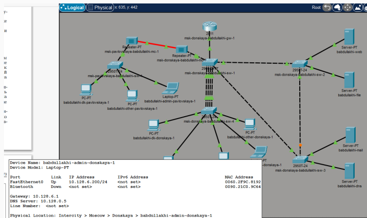
Рис. 1: Топология сети
