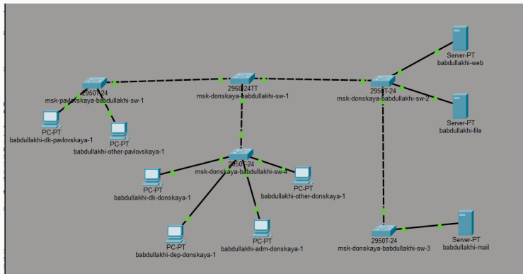
Рис. 1: Топология сети
