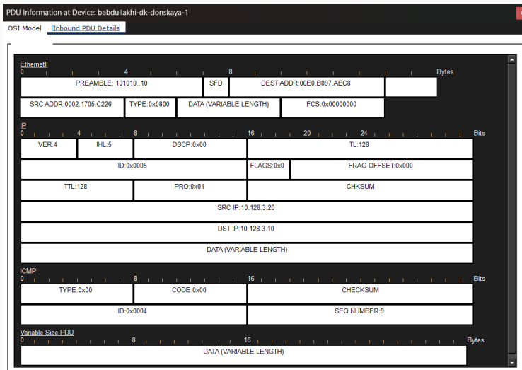
Рис. 11: Структура ICMP-пакета
