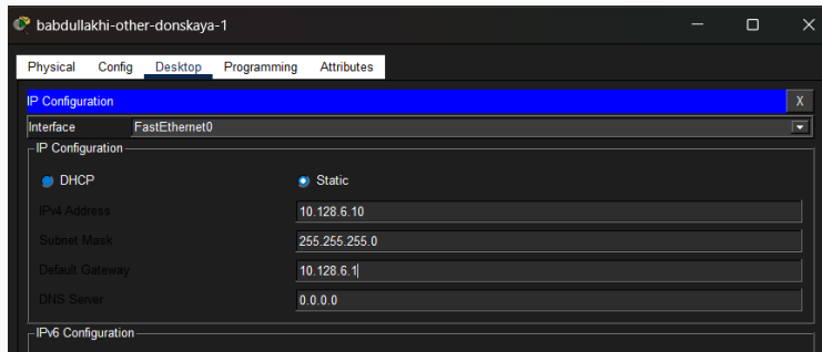
Рис. 8: Настройка IP ПК
