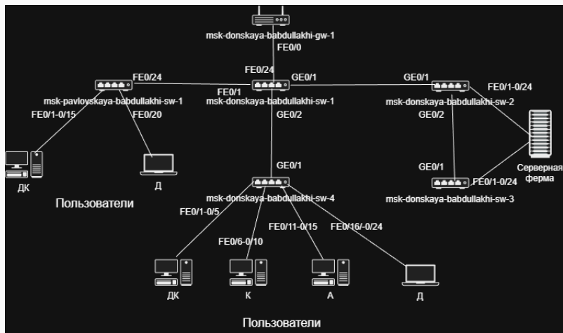
Рис. 1: Схема L1
