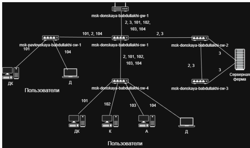
Рис. 2: Схема L2
