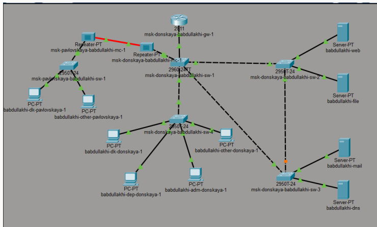
Рис. 1: Резервное соединение
