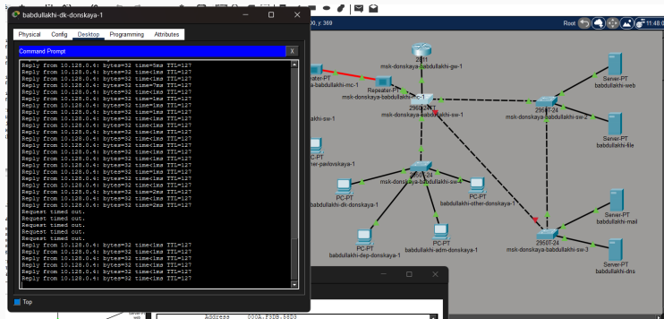
Рис. 7: STP отказ
