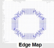
Edge Map
