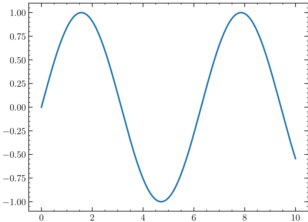
Sine Function
