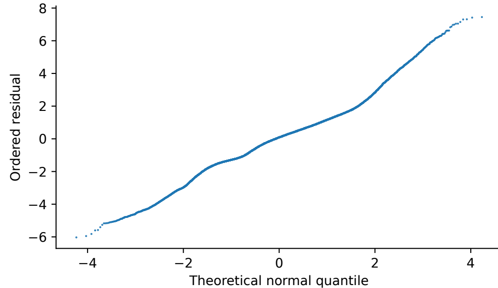
R0c normal Q-Q
