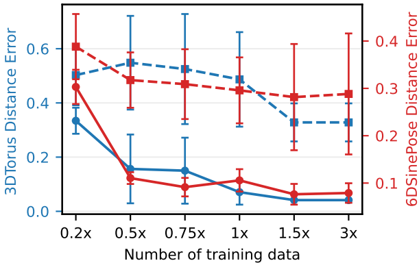
—●— 3DTorus - ONCL (Ours) —●— 6DSinePose - ONCL (Ours) —■— 3DTorus - ECoMaNN —■— 6DSinePose - ECoMaNN
