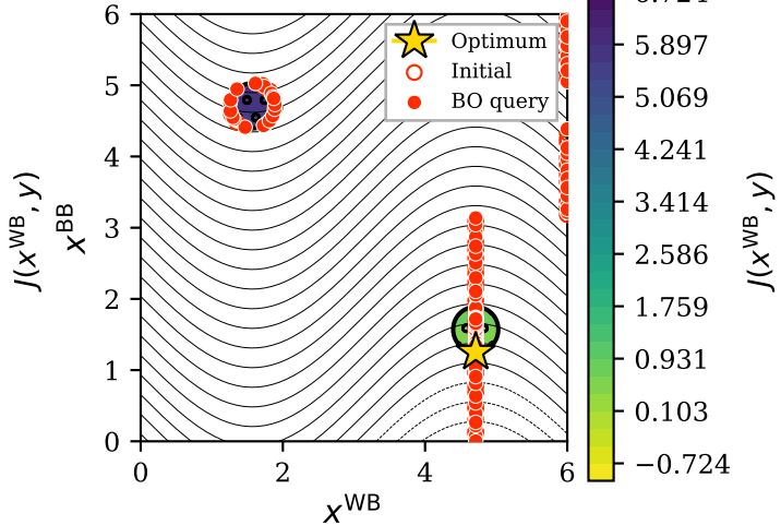
Bilevel BO
