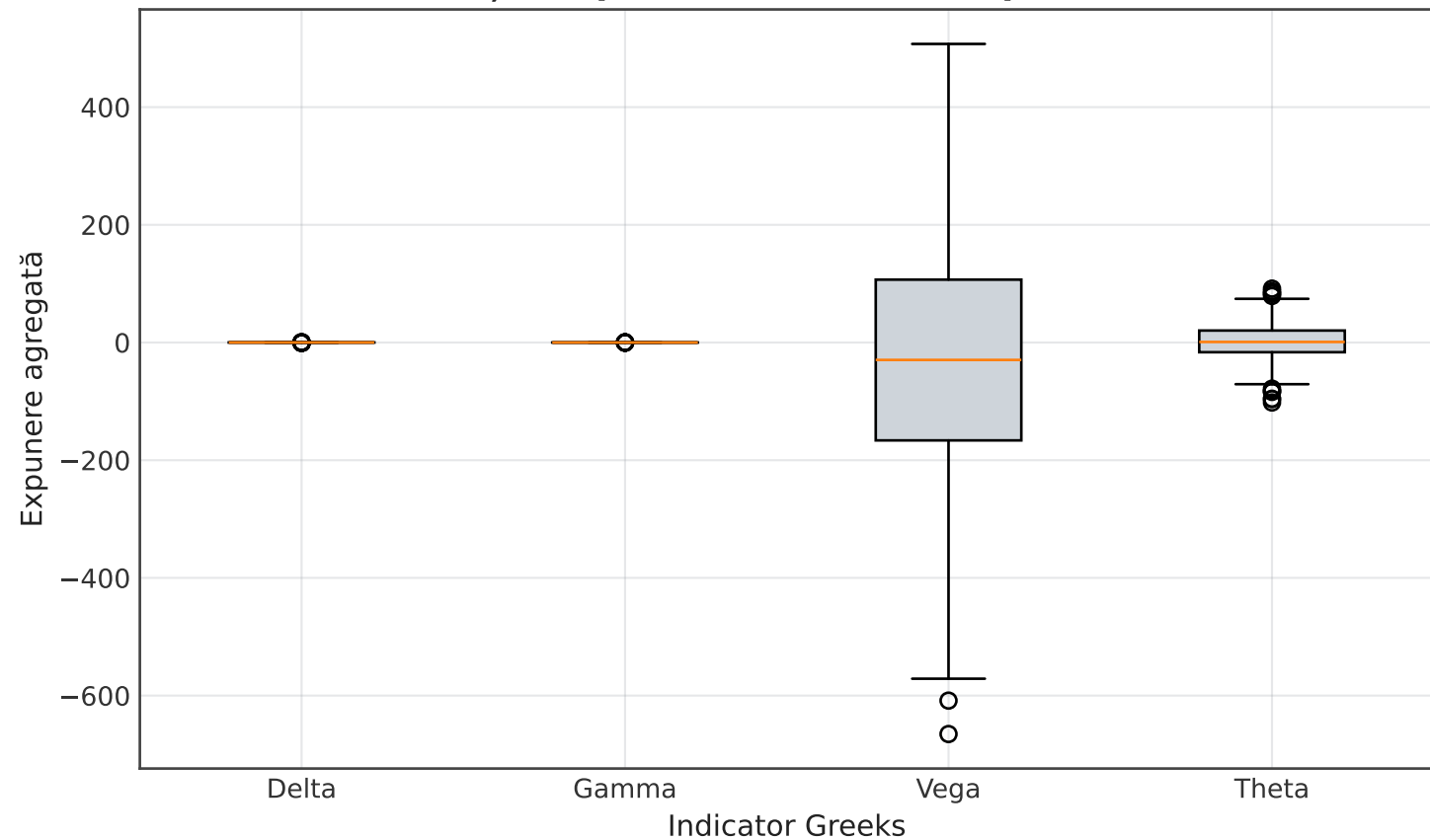
Distribuția expunerilor Greeks ale portofoliului
