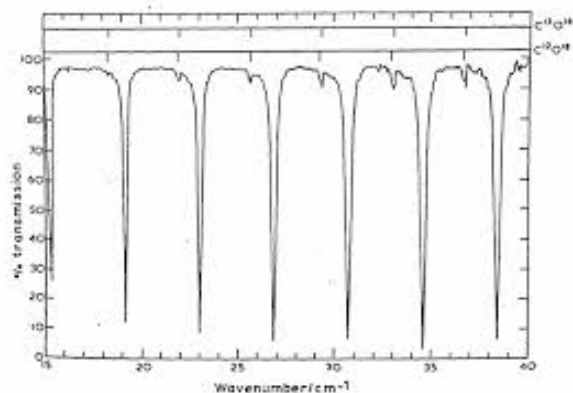
Figure 1: Spettro rotazionale
