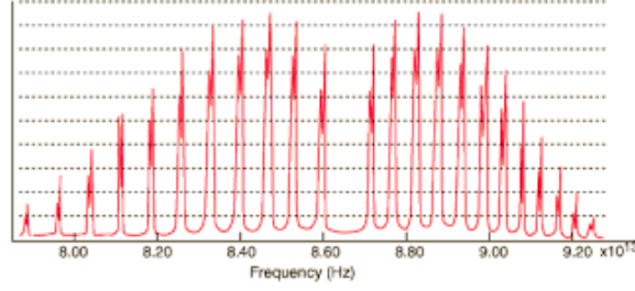
Figure 2: Spettro rotovibrazionale
