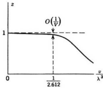
Figure 2: Z soluzione di (4.4.36)
