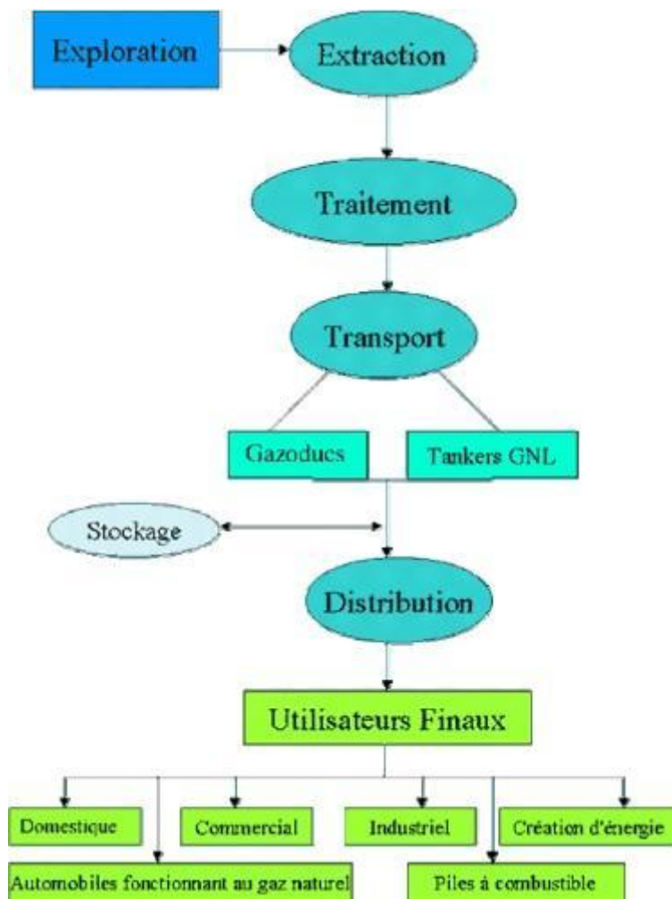
Principales étapes du traitement du gaz naturel.
