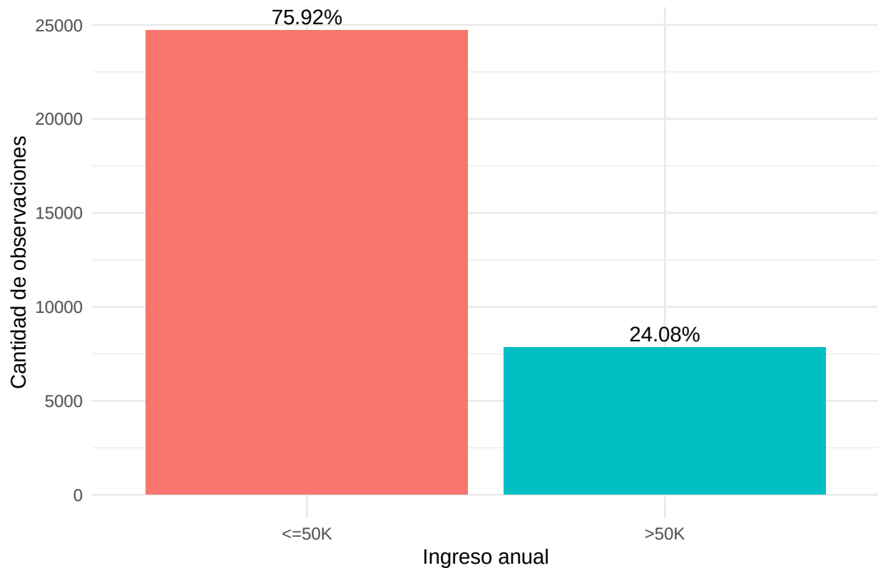
Distribución de la variable objetivo
