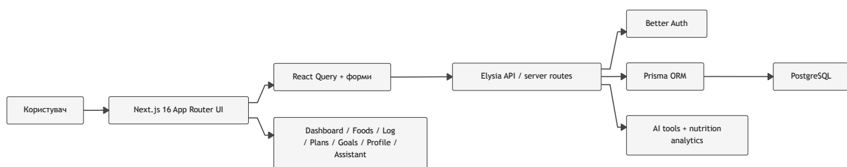
Figure 2: Mermaid-діаграма загальної архітектури NutriAI.
