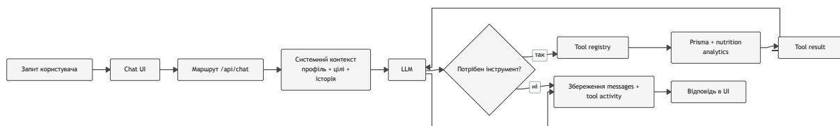
Figure 3: Mermaid-діаграма обробки AI-запиту в NutriAI.
