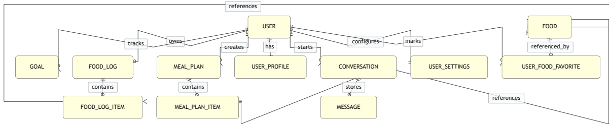
Figure 1: ER-діаграма основних сутностей NutriAI на основі Prisma-схеми.
