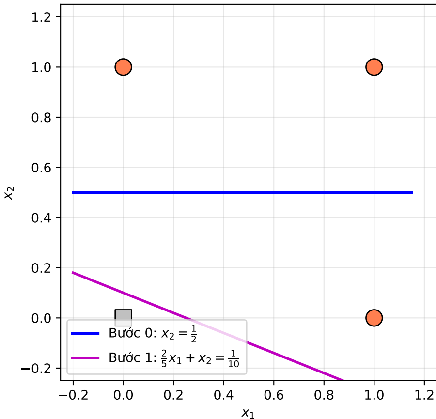
Perceptron GD batch, \rho = 0,4
