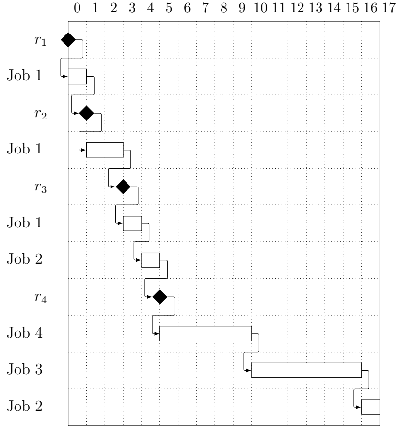
Hình 2.9: Sơ đồ Gantt ngắt quãng của phương án J_2^{(3)} .
