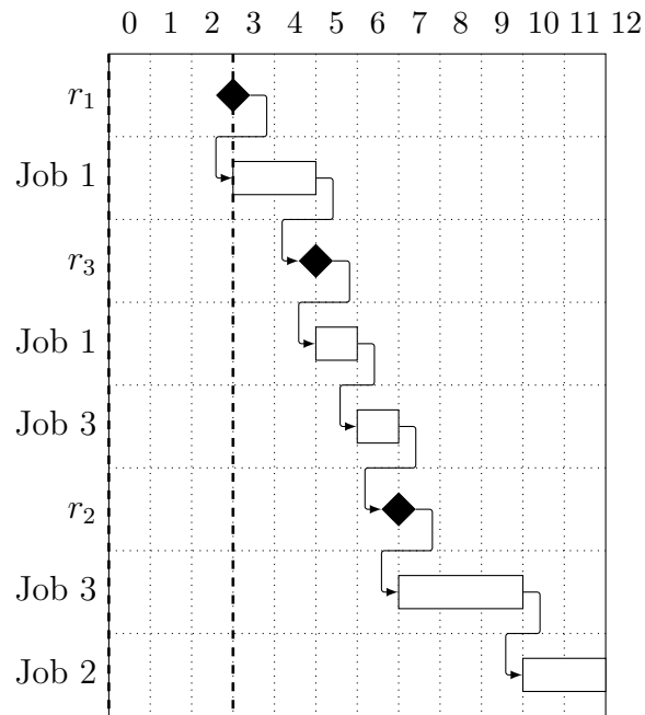
Hình 2.10: Sơ đồ Gantt không ngắt quãng của phương án J_0^{(1)} .
