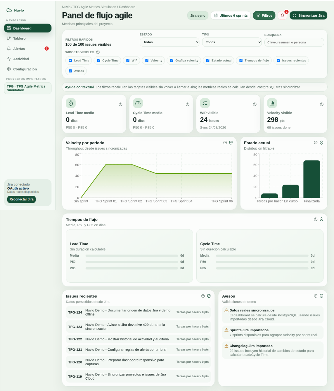
Figura A.3: Filtros rápidos y configuración de widgets
