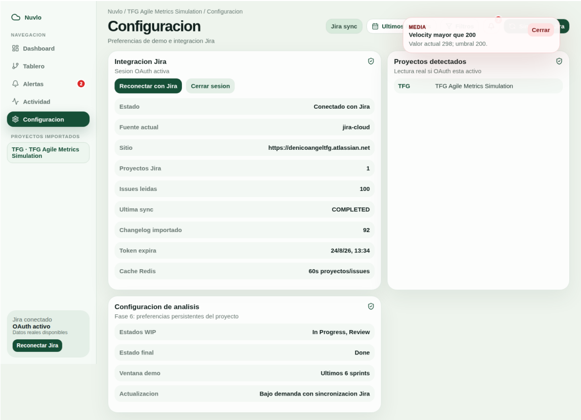
Figura A.7: Configuración y estado de conexión con Jira
