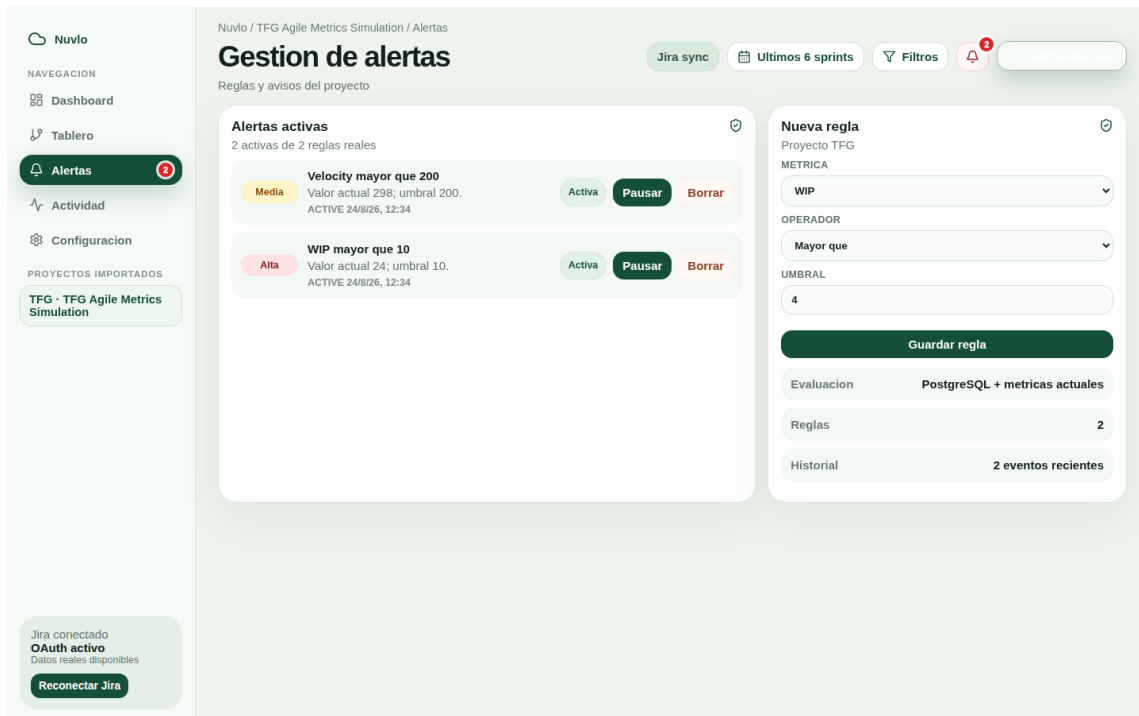
Figura A.5: Gestión de alertas por umbral
