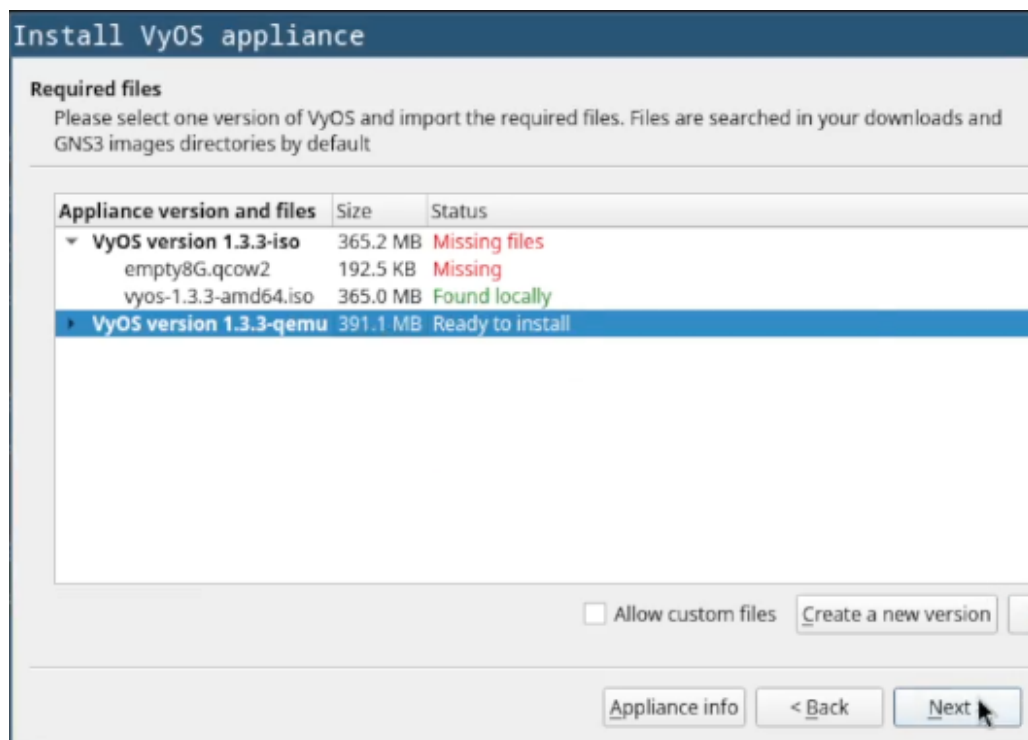
Рис. 12: Выбор установочного файла VyOS.
