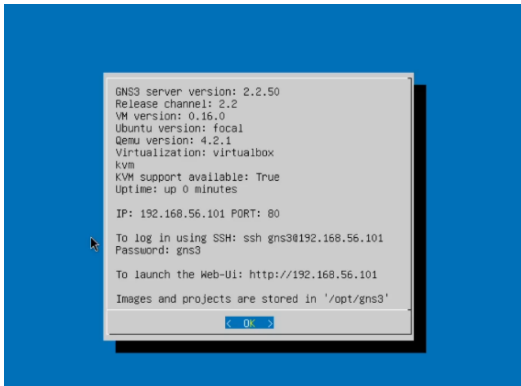
Рис. 6: Интерфейс GNS3 VM.
