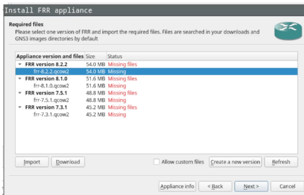
Рис. 10: Выбор версии установки FRR.
