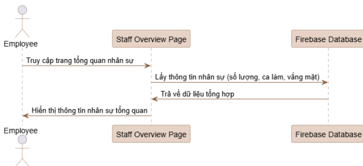
Hình 52: Biểu đồ tuần tự chức năng xem tổng quan nhân sự
