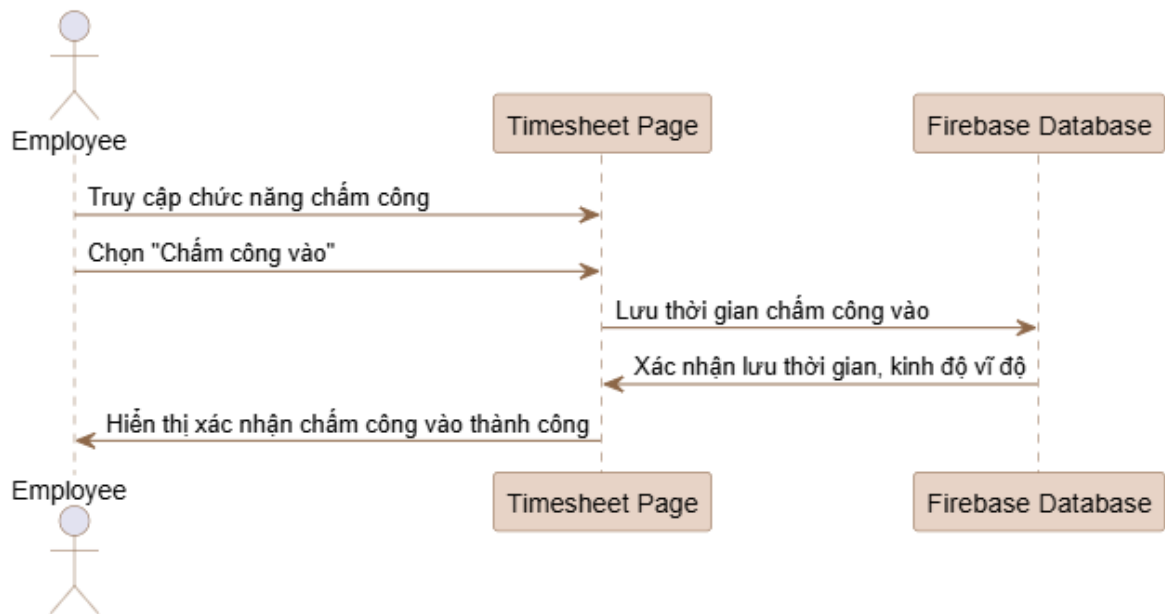
Hình 47: Biểu đồ tuần tự chức năng chấm công vào
