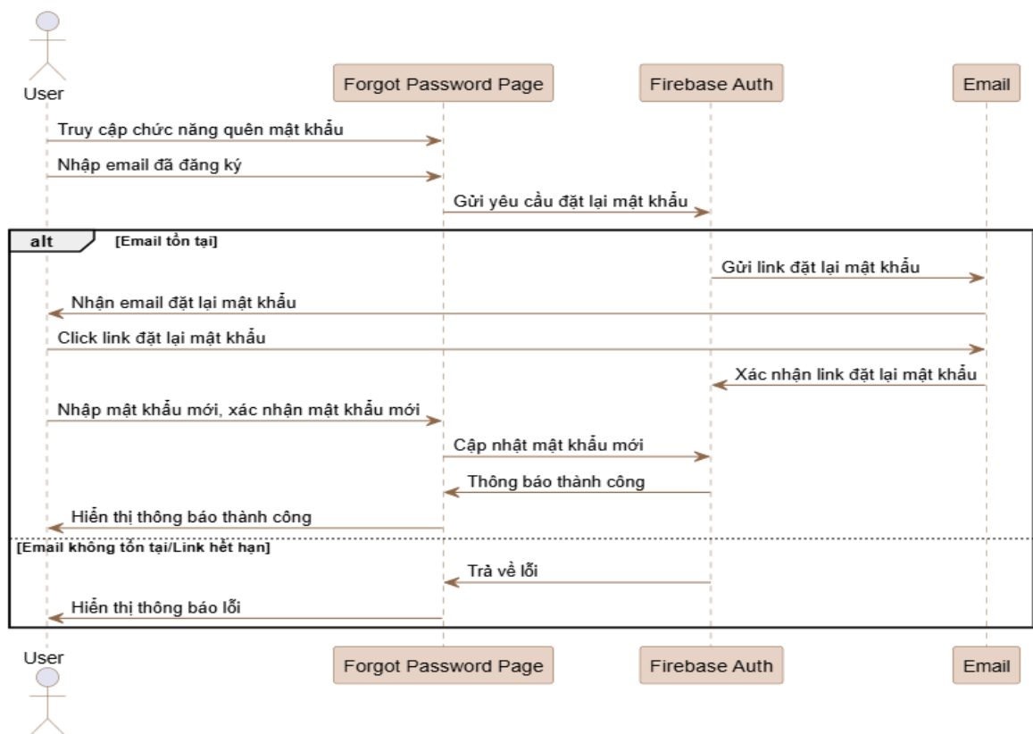
Hình 14: Biểu đồ tuần tự chức năng quên mật khẩu
