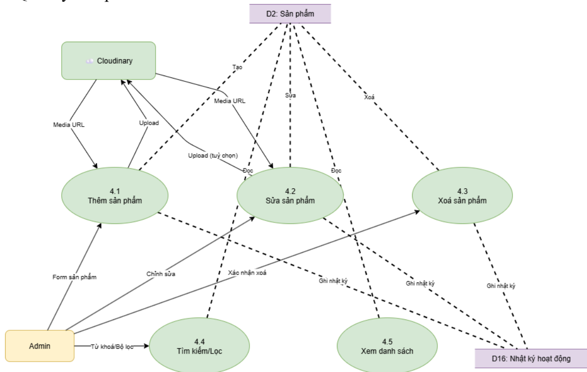
Hình 70: DFD cấp 2 Chi tiết tiến trình quản lý sản phẩm của Âm Coffee & Cake
