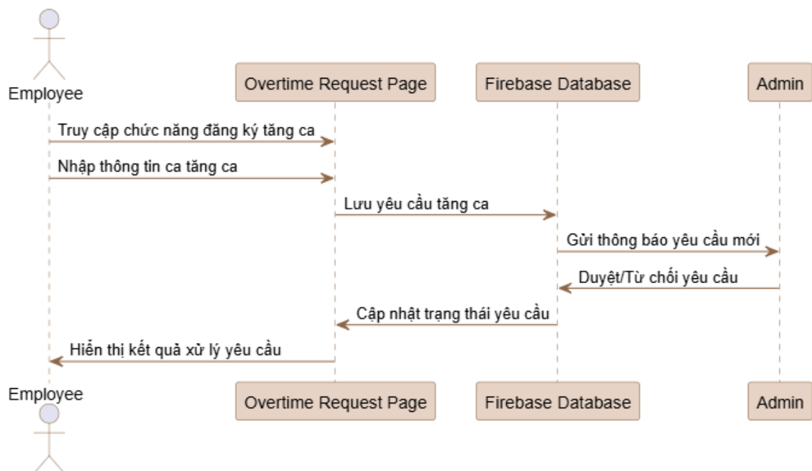
Hình 50: Biểu đồ tuần tự chức năng đăng ký tăng ca
