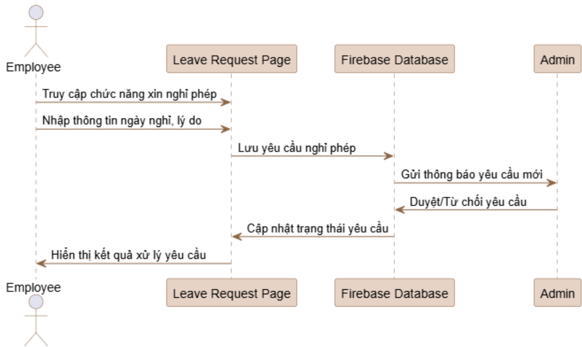
Hình 49: Biểu đồ tuần tự chức năng xin nghỉ phép
