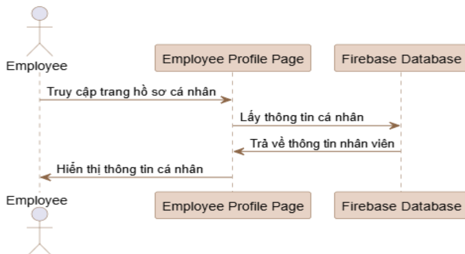
Hình 44: Biểu đồ tuần tự chức quản lý hồ sơ cá nhân
