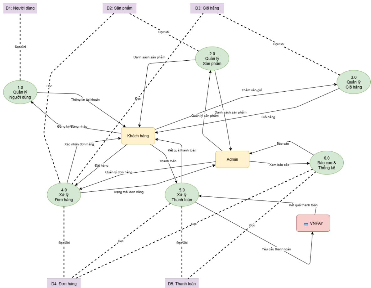
Hình 55: DFD cấp 1 phân rã của hệ thống bán hàng trực tuyến của Âm Coffee & Cake
