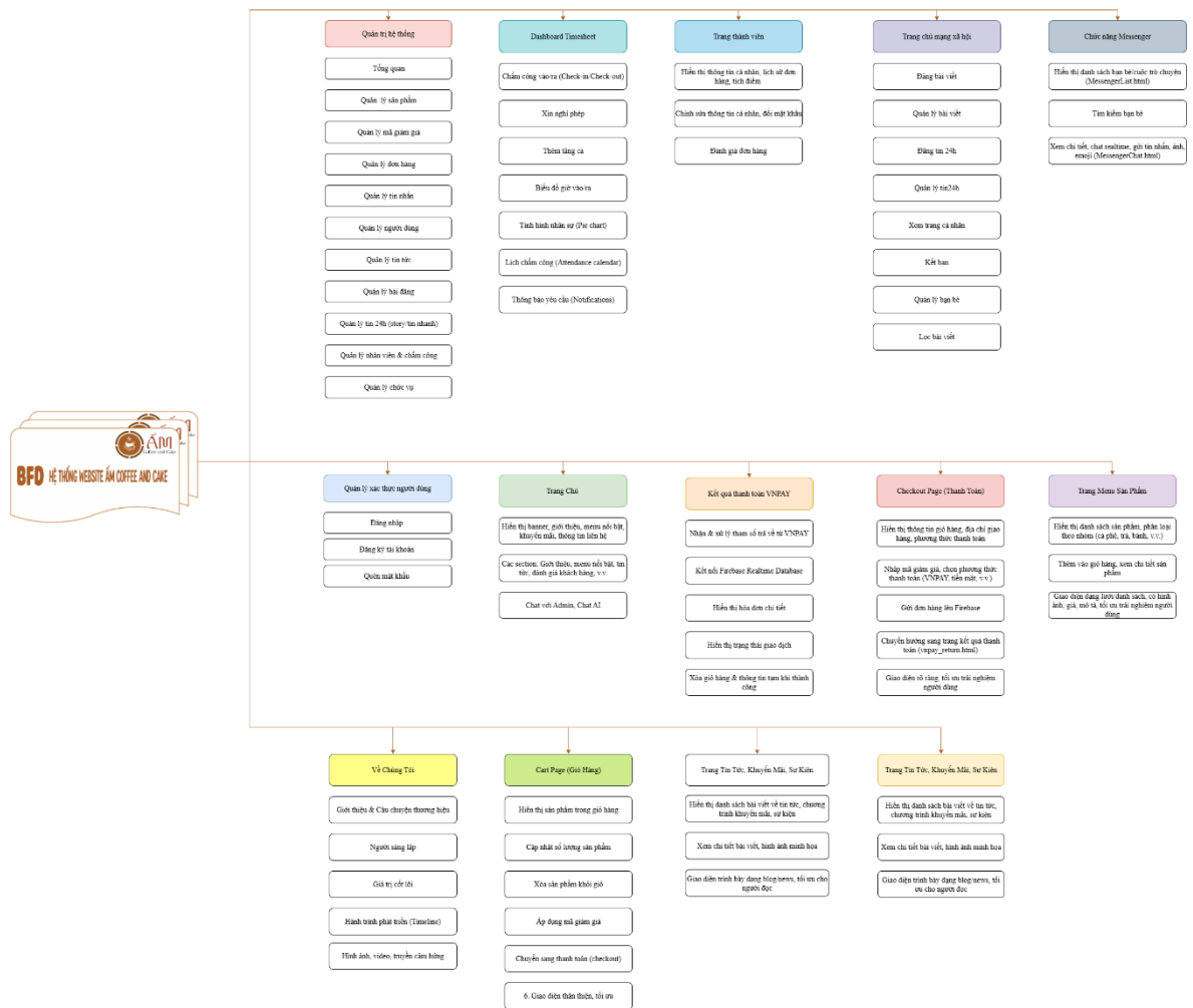
Hình 11: Biểu đồ phân rã chức năng BFD của hệ Website thương mại điện tử Ấm Coffee and Cake
