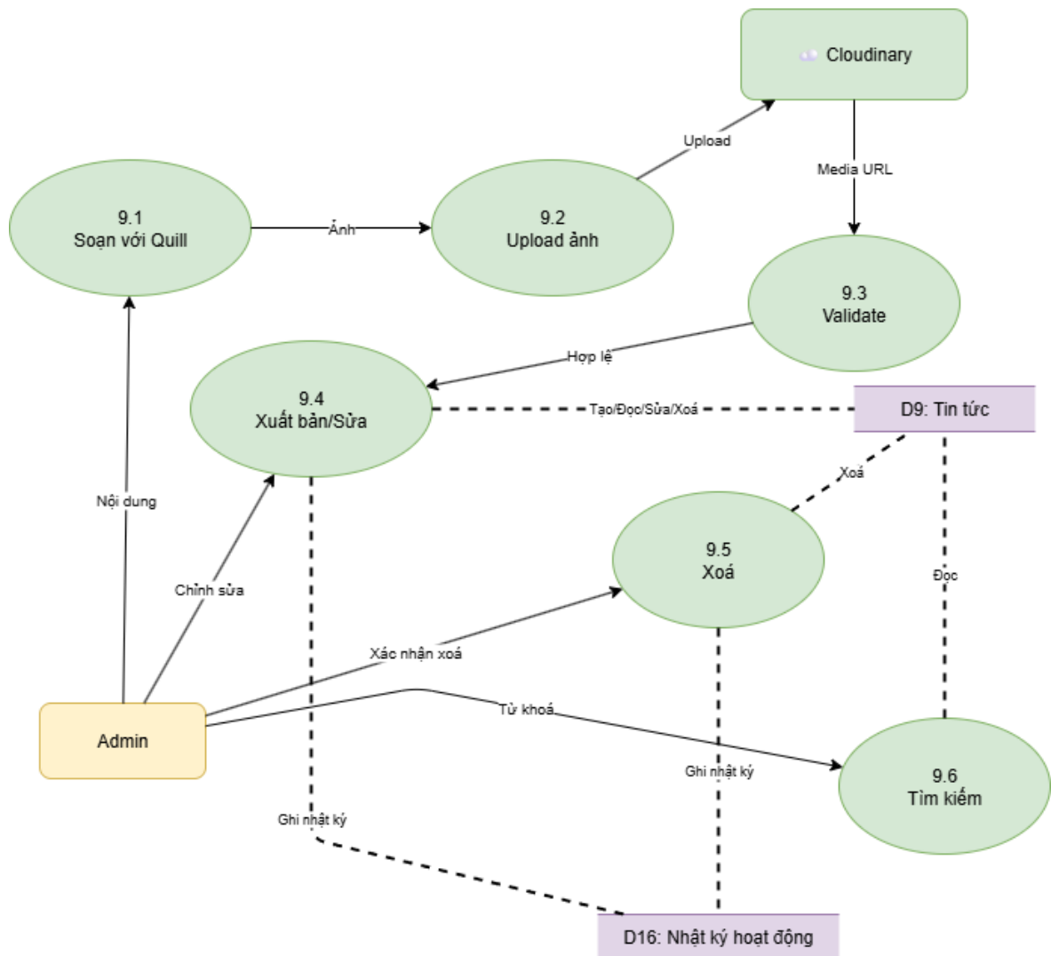
Hình 75: DFD cấp 2 Chi tiết tiến trình quản lý tin tức của Âm Coffee & Cake
