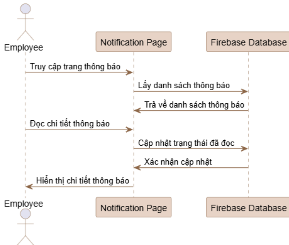
Hình 51: Biểu đồ tuần tự chức năng hiển thị thông báo
