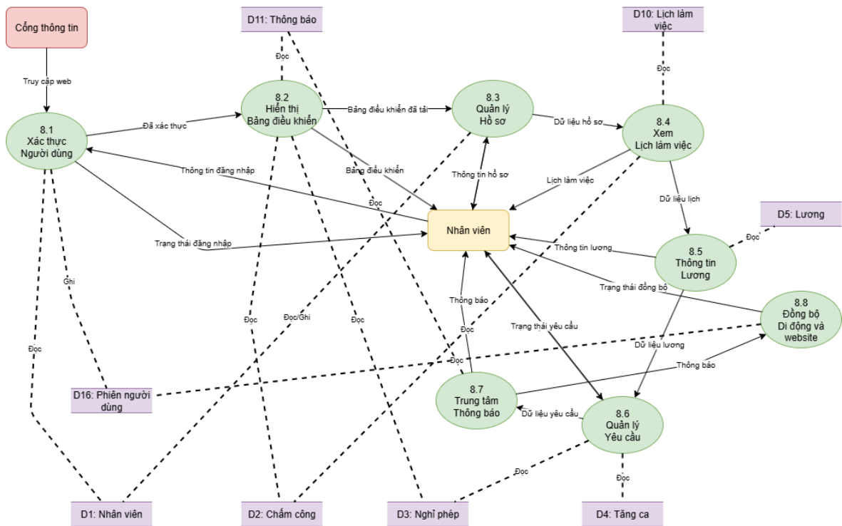
Hình 66: DFD cấp 2 Chi tiết tiến trình Chi tiết tiến trình Cổng thông tin nhân viên trực tuyến của Âm Coffee & Cake
