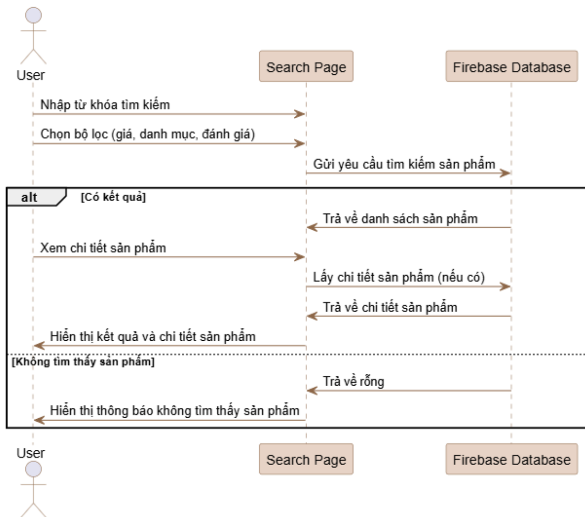
Hình 20: Biểu đồ tuần tự chức năng tìm kiếm sản phẩm
