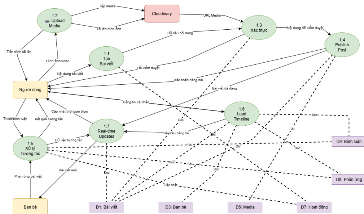
Hình 59: DFD cấp 2 Chi tiết tiến trình quản lý Bảng tin trực tuyến của Âm Coffee & Cake
