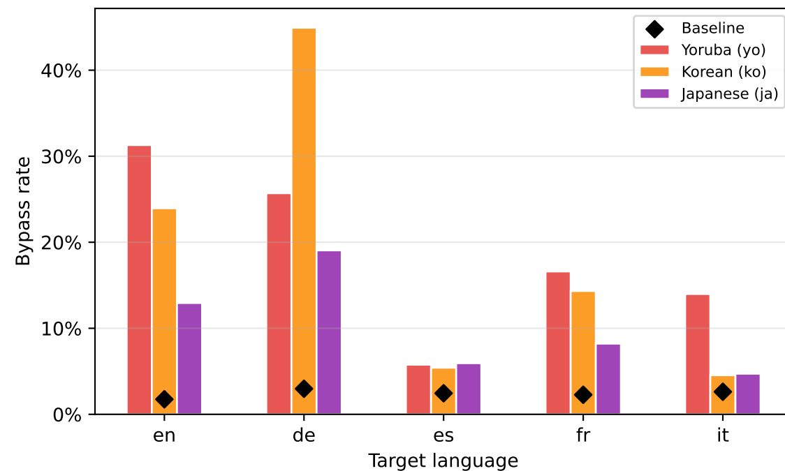
LLaMA-3.1-8B \alpha=20.0, k^*=28
