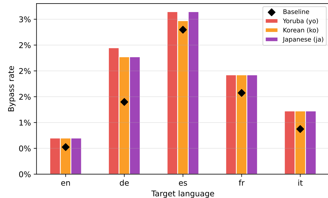
Gemma-2-9B \alpha=5.0, k^*=35
