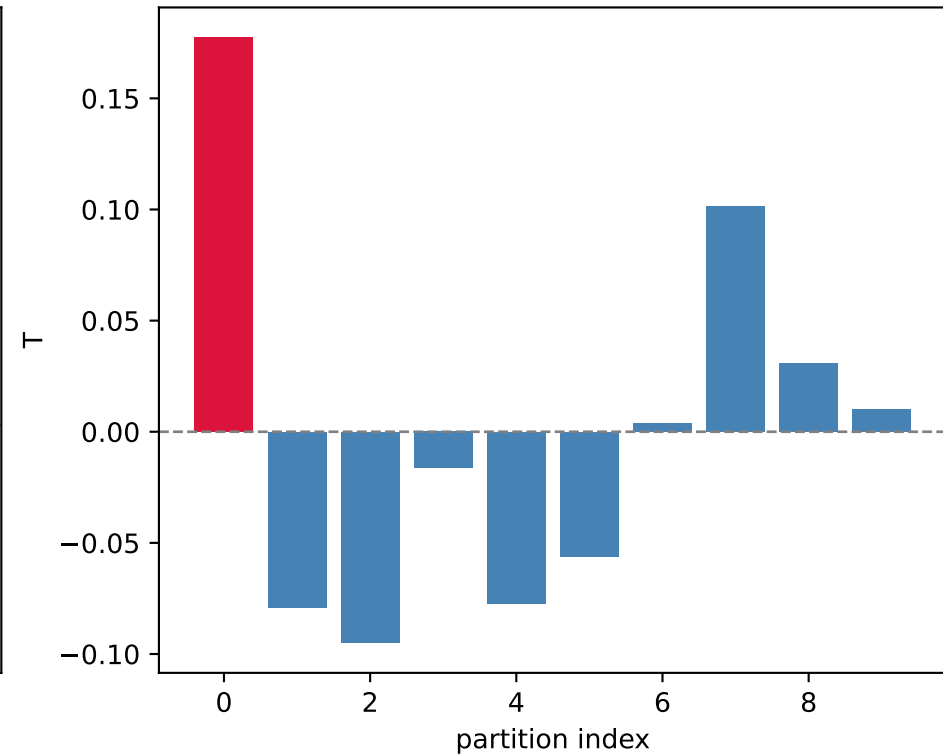
gemma-2-9b-it
