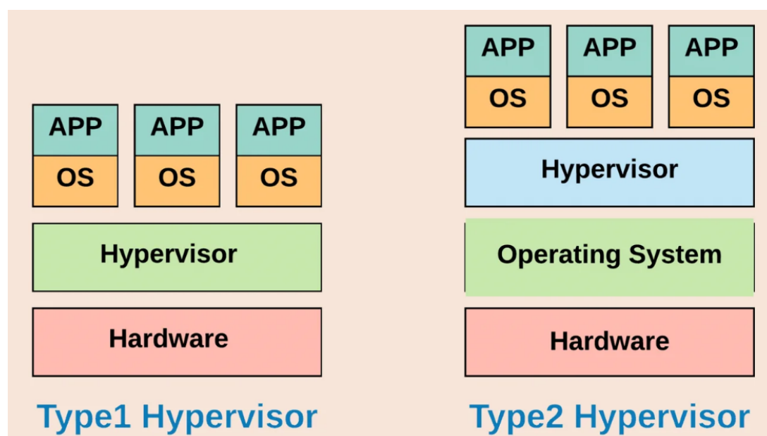
图 3.1 Type1 hypervisor 和 Type2 hypervisor 的架构对比
