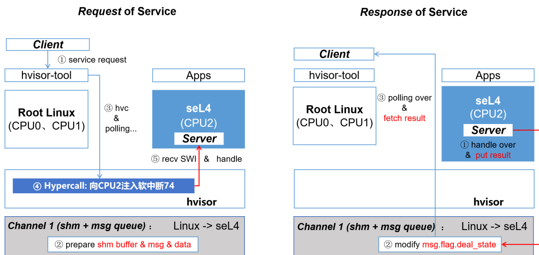
图 7.4 roo linux 与 seL4 间一次服务的请求和响应
