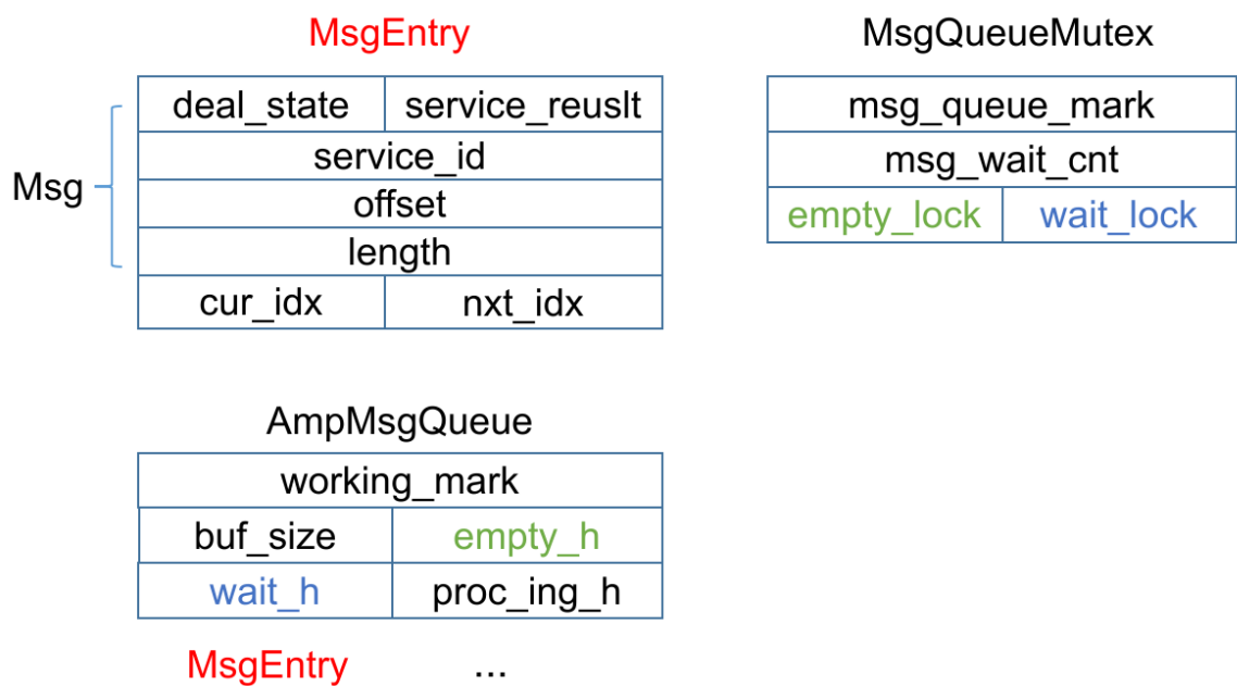
图 7.6 消息队列中重要的数据结构
