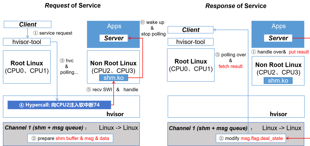
图 7.3 roo linux 与 non root 间一次服务的请求和响应
