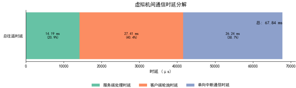
图 9.24 HyperAMP 跨虚拟机通信性能测试结果
