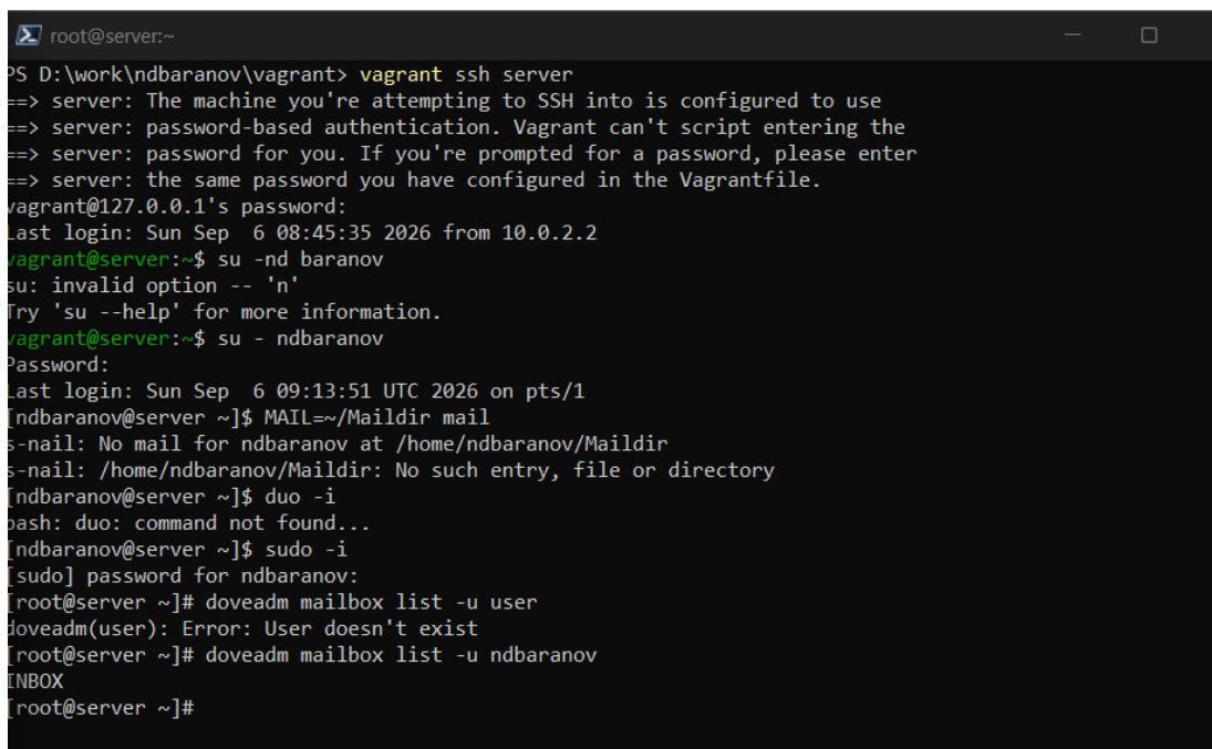
Рисунок 4.4: Создание структуры Maildir
